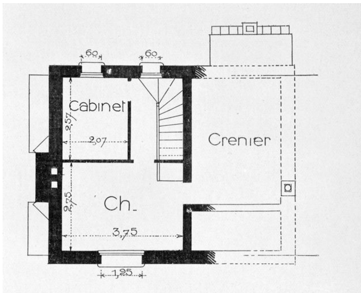
Plan de l'étage (AD Somme ; 1 J 3584/11).
