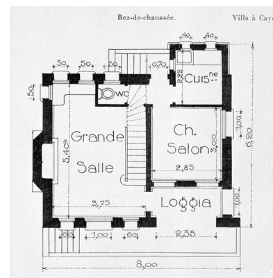
Plan du rez-de-chaussée (AD Somme ; 1 J 3584/11). Repro. Marie-Laure Monnehay-Vulliet IVR22_20038000340XB
