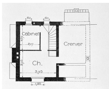
Plan de l'étage (AD Somme ; 1 J 3584/11).
