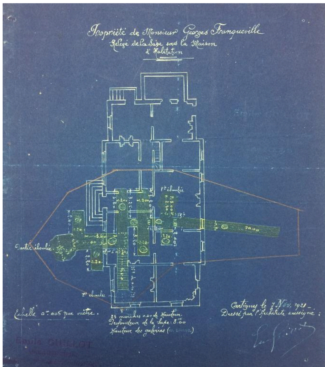
[Cartigny]. Propriété de M. Georges Franqueville. Relevé de la sape sous la maison d'habitation, par Emile Guillot, 1921 (AD Somme ; 10R 286).
