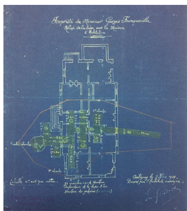
[Cartigny]. Propriété de M. Georges Franqueville. Relevé de la sape sous la maison d'habitation, par Emile Guillot, 1921 (AD Somme ; 10R 286). Phot. Isabelle Barbedor IVR32_20178005218NUCA
