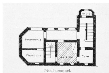
Plan du sous-sol, Raoul Brandon (AD Somme). Repro. Marie- Laure Monnehay-Vulliet IVR22_20038000333XB
