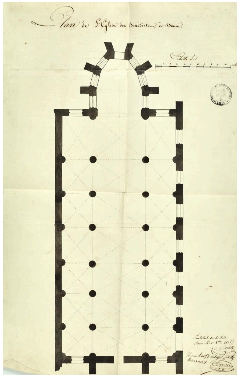
Plan de l'église des bénédictins à Douai. Daté et signé par l'architecte communal (signature illisible), le 8 octobre 1826. (AD Nord, 2O176/168).
