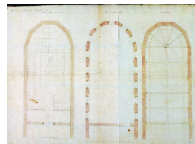
Douay, collegiale church. Plan au sol, coupe horizontale au niveau des baies et dessin de la voûte. Dessin d'Augustus Pugin ni daté ni signé, vers 1840. (AC Douai, 767W21). Phot. Pierre Thibaut IVR32_20225900429NUCA
