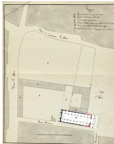
Plan avec le projet de modification de plan et d'orientation de la chapelle, vers 1815. Retombe du plan dressant l'état de l'existant. (AC Douai, 1P38). Phot. Pierre Thibaut IVR32_20225900416NUCA
