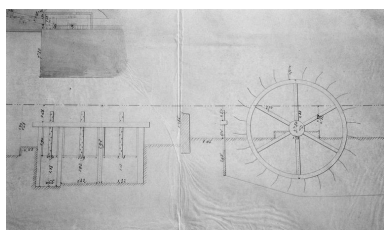
Élévation détaillée de profil du moulin de Froisselle, 1867 (AD Oise ; 7 Sp 223). Phot. Bertrand Fournier IVR22_20006000490ZB
