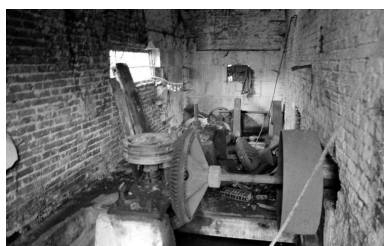
Intérieur de la cage du moulin abritant le mécanisme de transmission. Phot. Benoît Dufournier IVR22_19936000020Z
