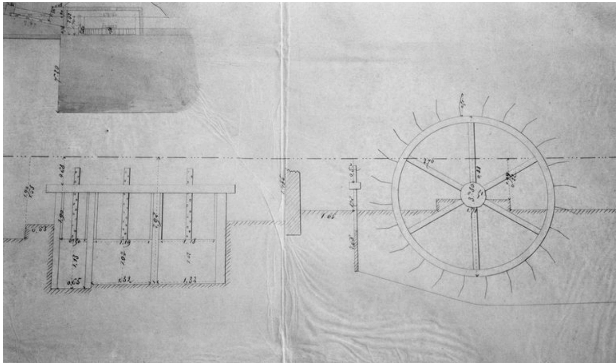
Elévation détaillée de profil du moulin de Froisselle, 1867 (AD Oise ; 7 Sp 223).
