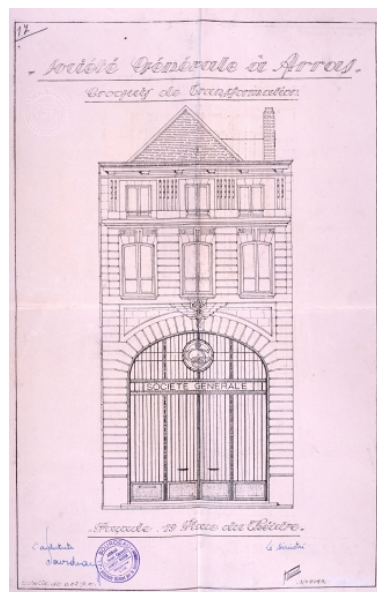
Croquis de transformation : façade, par Jean Sourdeau architecte, s. d. (AD Pas-de-Calais). Autr. Jean Sourdeau, Phot. Thibaut Pierre (reproduction) IVR31_20096200118XA
