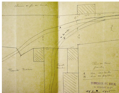
Projet d'établissement d'une voie aiguillée pour raccorder les nouveaux bâtiments de la verrerie à la voie existante, plan, 1906 (AC Creil ; 101 108). Repro. Clarisse Lorieux IVR22_20076005467NUCAB
