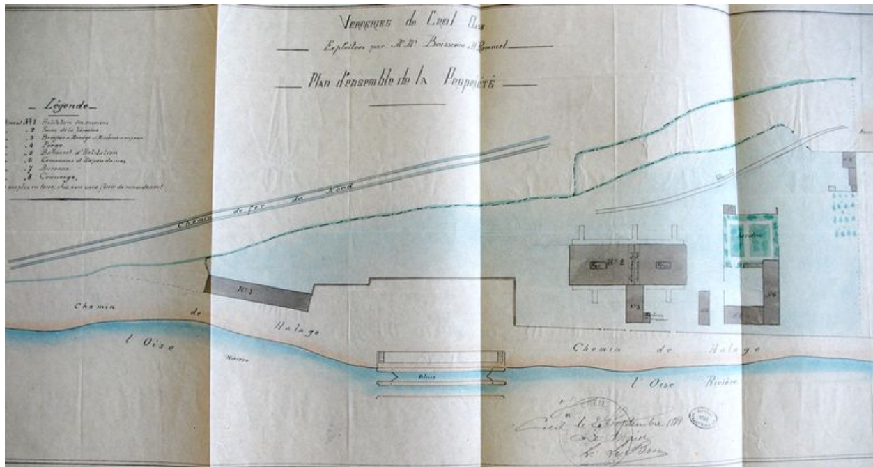
Plan de la verrerie Boissière et Rommel, 1888 (AD Oise ; 5Mp2455/1).
