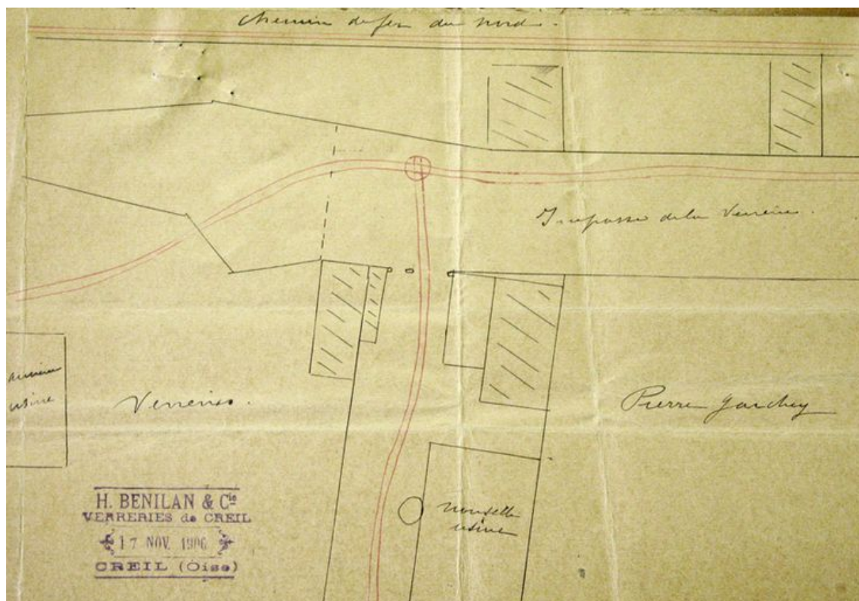
Plan de la plaque tournante réalisée en 1906 par les établissements Calvet, Aubagnac, Jeune et Gonnot (La Plaine Saint-Denis) pour le raccordement de la verrerie (AC Creil ; 1O1 108).
