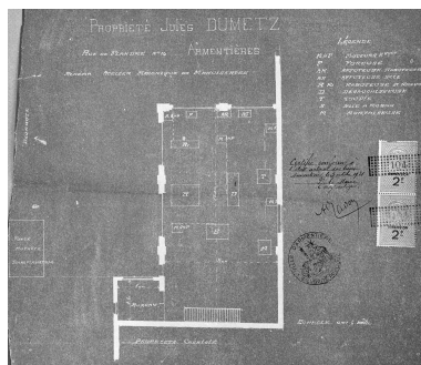
Installation de la scierie Jules Dumetz. Plan masse, 1921 (AD Nord ; M 41710347). Repro. Philippe Dapvril IVR31_19875902066X
