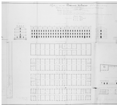
Bâtiment principal : plans, coupe, façade, 1859. A. Génie Vincennes, Boulogne, art. 8, section 1, carton 9. Repro. Philippe Dapvril IVR31_19946200776X
