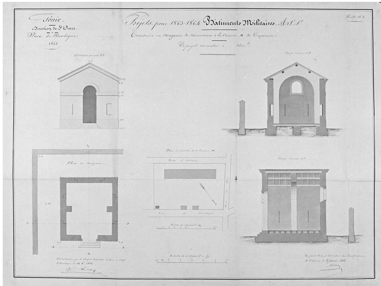
Magasin de munitions, plans, coupes, façades. A. Génie Vincennes, Boulogne, art. 8, section 1, carton 9.
