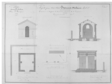
Magasin de munitions, plans, coupes, façades. A. Génie Vincennes, Boulogne, art. 8, section 1, carton 9. Repro. Philippe Dapvril IVR31_19946200777X
