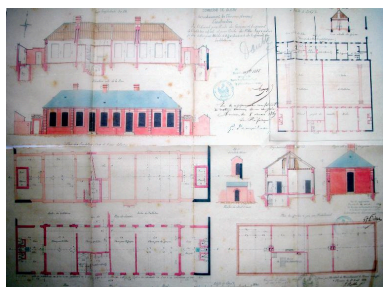
Plans, coupes et élévations de la mairie-école, J. Robbe (architecte), 31 août 1868 (AD Somme ; 99 O 1181).
