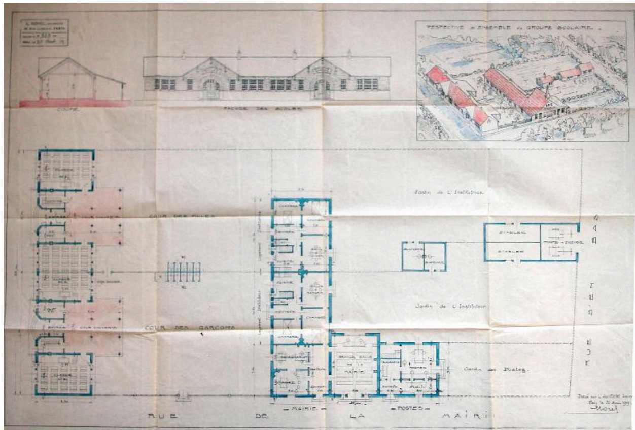
Plan, coupe, élévation et perspective d'ensemble, L. Sorel (architecte), 20 août 1919 (AD Somme ; 99 O 1181).
