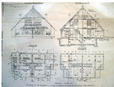
Cité de la Canardière. Type de maison à 2 logements de 4 pièces (pl. 27). La construction Moderne, n° 11, 12 décembre 1926 Phot. Barbedor Isabelle IVR22_20048010760NUCA
