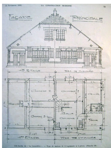
Cité de la Canardière. Type de maison à 2 logements de 4 pièces (pl. 28). La construction Moderne, n° 11, 12 décembre 1926 Phot. Barbedor Isabelle
