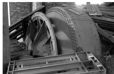
Broyeur à galets. Phot. Benoît Dufournier IVR22_19888000287Z
