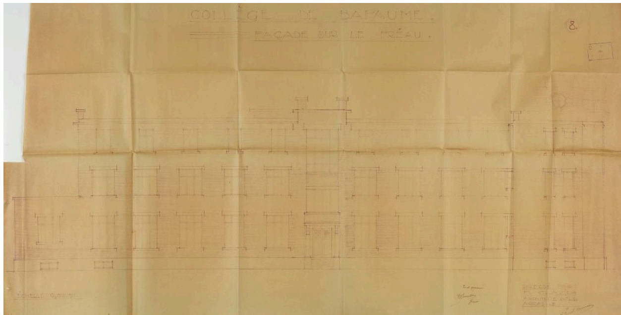
Collège de Bapaume. Façade sur le préau - 8. Plan à l'échelle 0,02 P.M., signé par le maître d'ouvrage et Paul Clavier (architecte), sans date. (AD Pas de Calais, 10R9/100, dossier n°1520).
