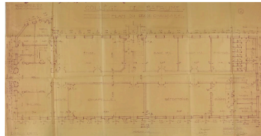
Collège de Bapaume. Plan du rez-de-chaussée - 2. Plan à l'échelle 0,02 P.M., signé par le maître d'ouvrage et Paul Clavier (architecte), sans date. (AD Pas de Calais, 10R9/100, dossier n°1520). Phot. Pierre Thibaut IVR32_20216200218NUCA
