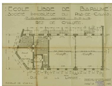
École libre de Bapaume - Société Immobilière du Pas-de-Calais. P. Clavier architecte D.P.L.G. : rez-de-chaussée. Signé et daté par l'architecte le 21 septembre 1922. (AD Pas-de-Calais, 10R9/44, dossier n°654). Phot. Pierre Thibaut IVR32_20216200354NUCA
