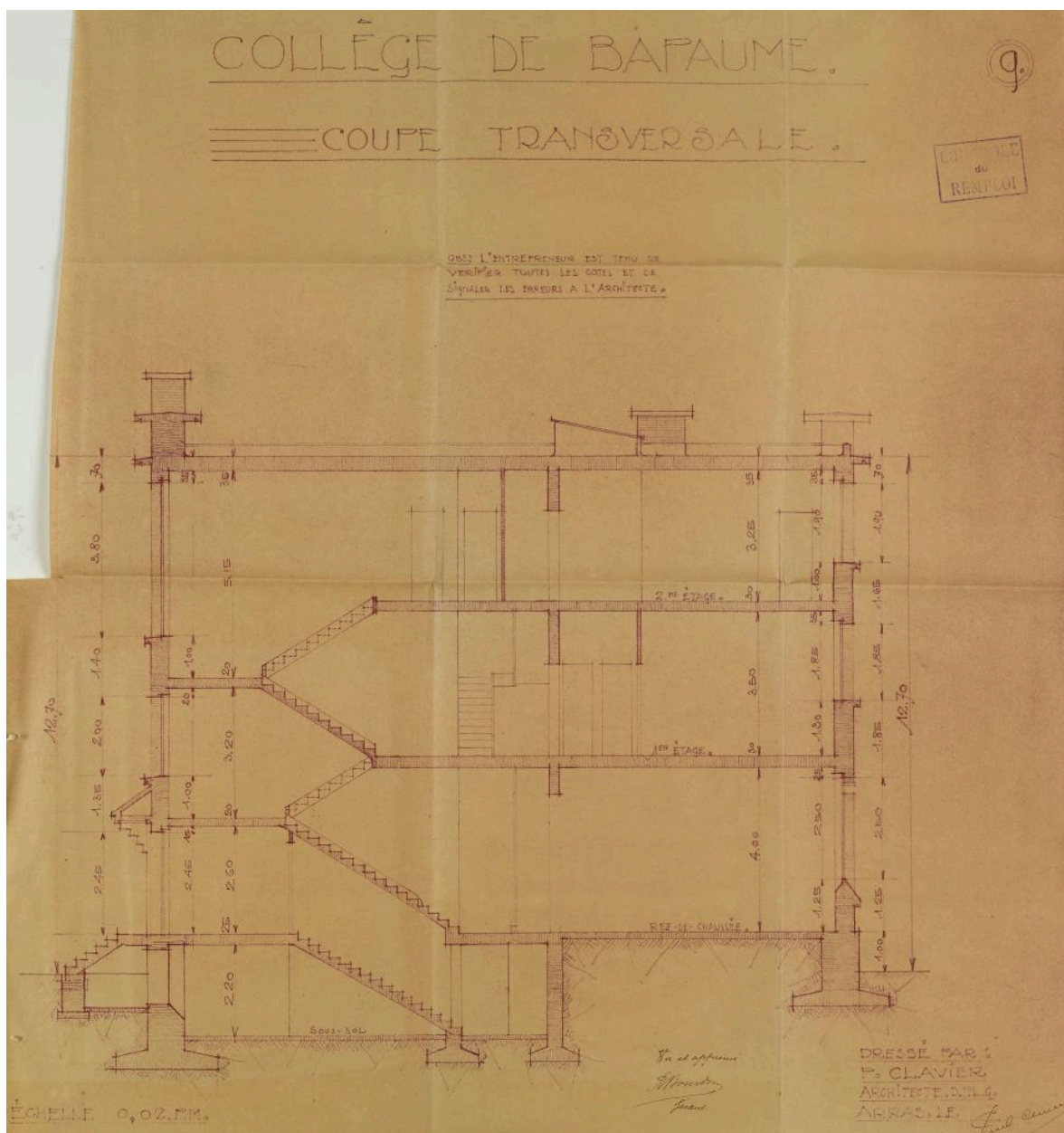
Collège de Bapaume. Coupe transversale - 9. Plan à l'échelle 0,02 P.M., signé par le maitre d'ouvrage et Paul Clavier (architecte), sans date. (AD Pas de Calais, 10R9/100, dossier n°1520).
