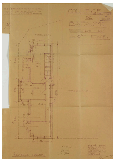
Collège de Bapaume. Plan du 3ème étage - 10. Plan à l'échelle 0,02 P.M., signé par le maître d'ouvrage et Paul Clavier (architecte), sans date. (AD Pas de Calais, 10R9/100, dossier n°1520).
