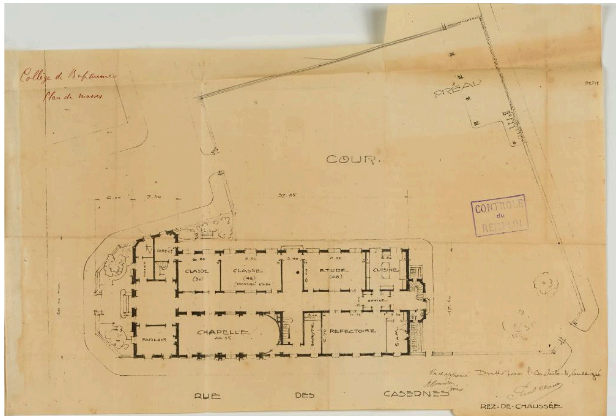
Collège de Bapaume. Plan de masse. Signé par le maître d'ouvrage et Eugène Rousseau (architecte), sans date. (AD Pas de Calais, 10R9/100, dossier n°1520).
