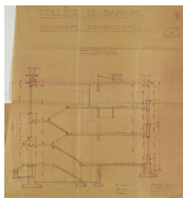
Collège de Bapaume. Coupe transversale - 9. Plan à l'échelle 0,02 P.M., signé par le maître d'ouvrage et Paul Clavier (architecte), sans date. (AD Pas de Calais, 10R9/100, dossier n°1520).
