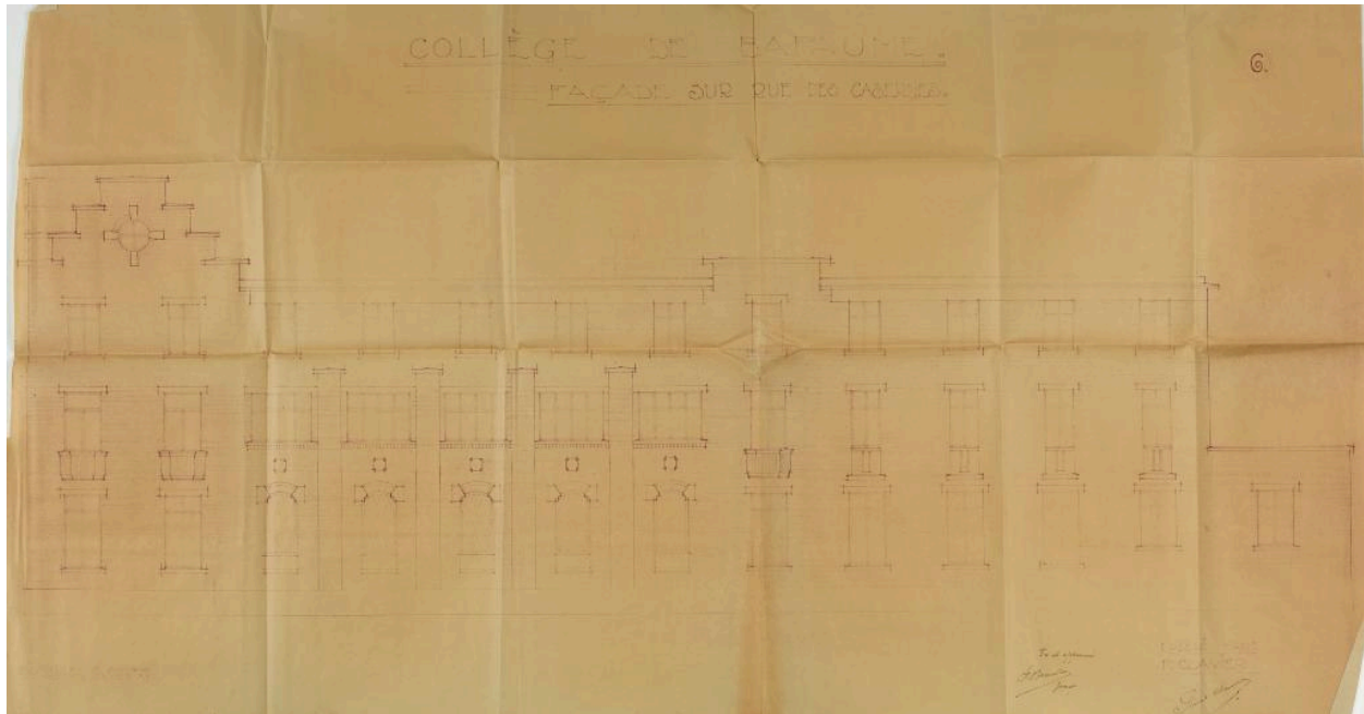
Collège de Bapaume. Façade sur rue des casernes - 6. Plan à l'échelle 0,02 P.M., signé par le maitre d'ouvrage et Paul Clavier (architecte), sans date. (AD Pas de Calais, 10R9/100, dossier n°1520).
