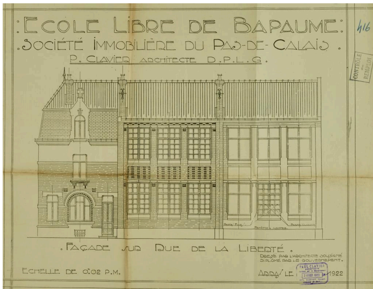
École libre de Bapaume - Société Immobilière du Pas-de-Calais. P. Clavier architecte D.P.L.G. : façade rue de la Liberté. Signé et daté par l'architecte le 21 septembre 1922. (AD Pas-de-Calais, 10R9/44, dossier n°654).
