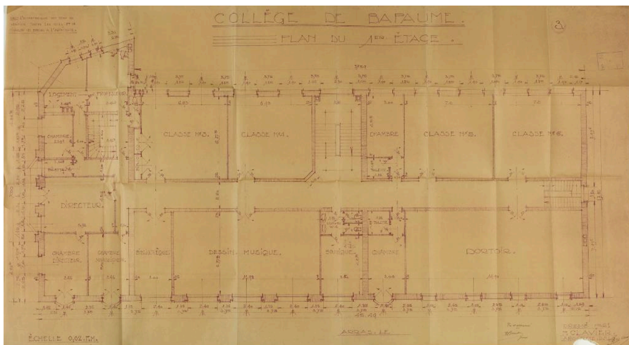
Collège de Bapaume. Plan du 1er étage - 3. Plan à l'échelle 0,02 P.M., signé par le maitre d'ouvrage et Paul Clavier (architecte), sans date. (AD Pas de Calais, 10R9/100, dossier n°1520).
