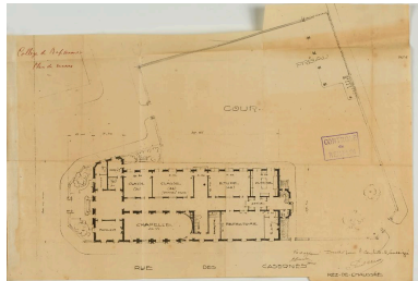
Collège de Bapaume. Plan de masse. Signé par le maître d'ouvrage et Eugène Rousseau (architecte), sans date. (AD Pas de Calais, 10R9/100, dossier n°1520). Phot. Pierre Thibaut IVR32_20216200216NUCA
