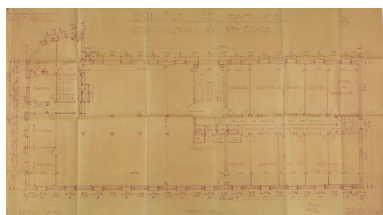
Collège de Bapaume. Plan du 2ème étage - 4. Plan à l'échelle 0,02 P.M., signé par le maître d'ouvrage et Paul Clavier (architecte), sans date. (AD Pas de Calais, 10R9/100, dossier n°1520). Phot. Pierre Thibaut IVR32_20216200220NUCA
