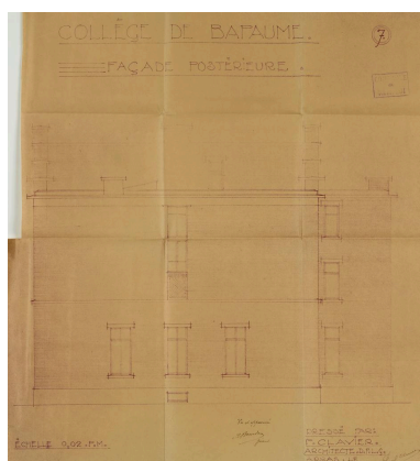
Collège de Bapaume. Façade postérieure - 7. Plan à l'échelle 0,02 P.M., signé par le maître d'ouvrage et Paul Clavier (architecte), sans date. (AD Pas de Calais, 10R9/100, dossier n°1520).
