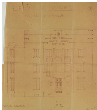
Collège de Bapaume. Façade de l'entrée - 5. Plan à l'échelle 0,02 P.M., signé par le maître d'ouvrage et Paul Clavier (architecte), sans date. (AD Pas de Calais, 10R9/100, dossier n°1520). Phot. Pierre Thibaut IVR32_20216200221NUCA
