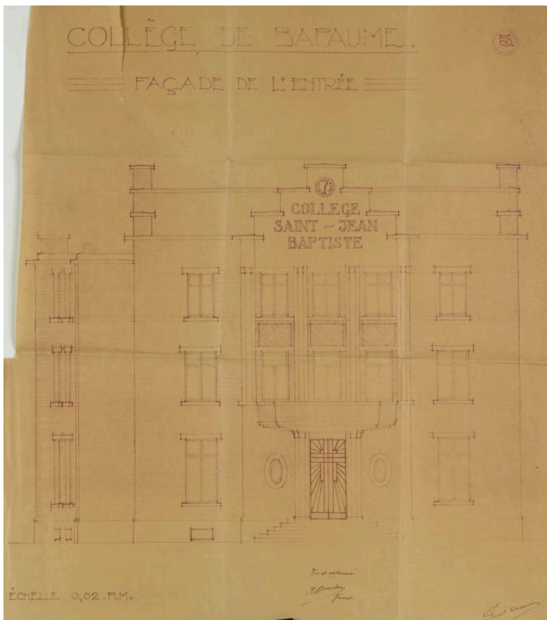
Collège de Bapaume. Façade de l'entrée - 5. Plan à l'échelle 0,02 P.M., signé par le maître d'ouvrage et Paul Clavier (architecte), sans date. (AD Pas de Calais, 10R9/100, dossier n°1520).
