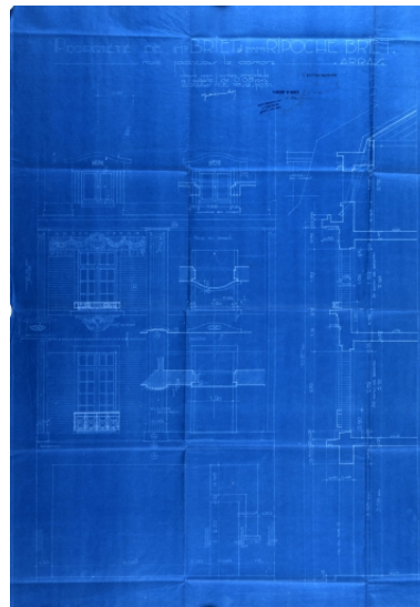
Propriété de M. Briet-Ripoche à Arras. Projet de construction : façade et coupe, par Wirton architecte, février 1931 (AD Pas-de-Calais). Autr. Julien Wirton, Phot. Thibaut Pierre (reproduction) IVR31_20096200130XA
