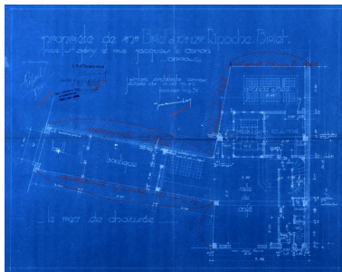
Propriété de M. Briet et MM. Ripoche-Briet à Arras. Projet de construction : plan du rez-de-chaussée, par Wirton architecte, janvier 1931 (AD Pas-de-Calais). Phot. Thibaut Pierre (reproduction), Phot. Julien Wirton IVR31_20096200132XA
