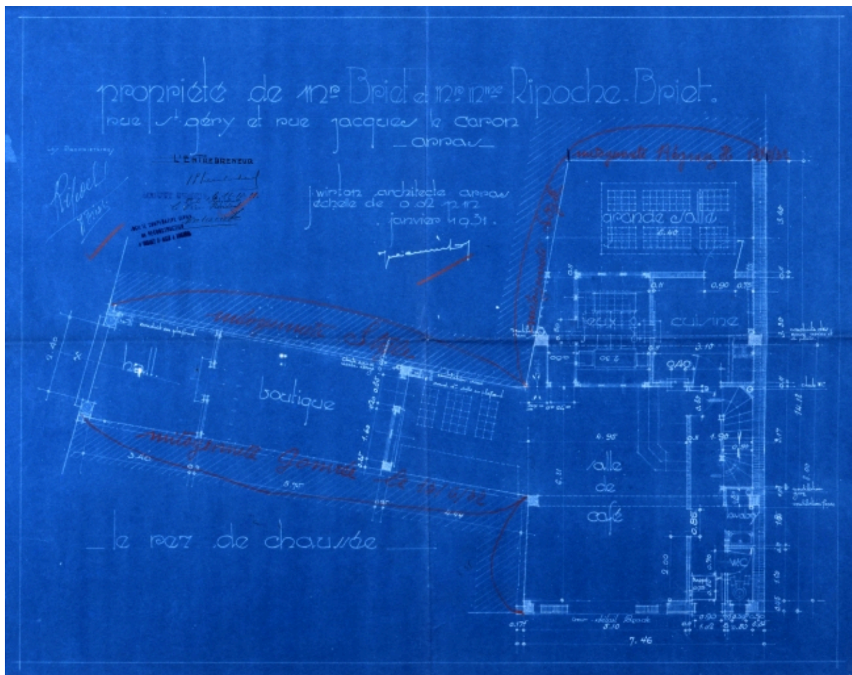
Propriété de M. Briet et MM. Ripoché-Briet à Arras. Projet de construction : plan du rez-de-chaussée, par Wirton architecte, janvier 1931 (AD Pas-de-Calais).
