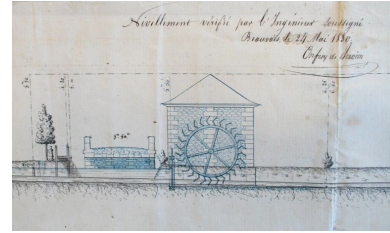
Profil modifié du moulin appartenant à Leroy-Beaucousin, 1830.
