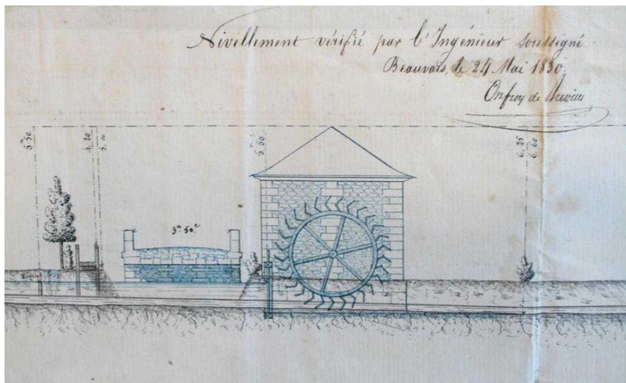
Profil modifié du moulin appartenant à Leroy-Beaucousin, 1830.
