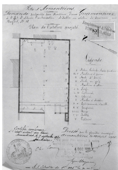
Pierre Guermontprez. Établissement d'un atelier de serrurerie, plan masse, 1920 (AD Nord ; M 41710317) Repro. Philippe Dapvril IVR31_19885901286X
