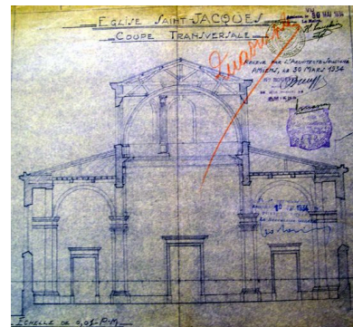
Coupe transversale, 1934 (AD Somme ; 99 O 303). Phot. Isabelle Barbedor, Phot. Georges Bouffet IVR22_20068010142NUCA
