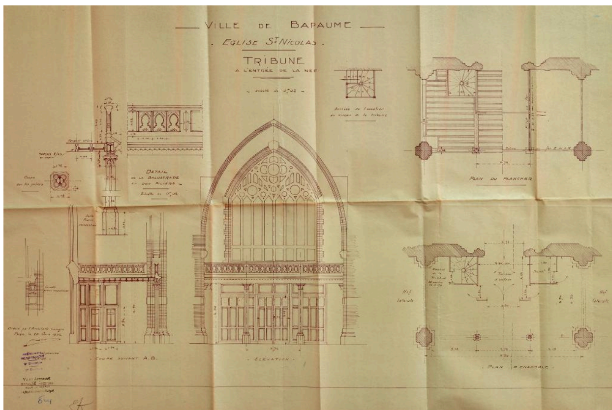
Ville de Bapaume - Église Saint-Nicolas - tribune à l'entrée de la nef : plan d'ensemble ; élévation ; coupe suivant AB ; détail de la balustrade et des piliers ; plan du plancher. Signé et daté, Eugène Bidard, le 25 juin 1932. (AD Pas-de-Calais, 2O609/6).
