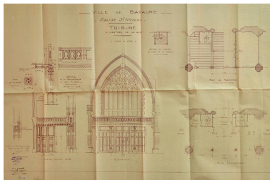
Ville de Bapaume - Église Saint- Nicolas - tribune à l'entrée de la nef : plan d'ensemble ; élévation ; coupe suivant AB ; détail de la balustrade et des piliers ; plan du plancher. Signé et daté, Eugène Bidard, le 25 juin 1932. (AD Pas-de-Calais, 2O609/6). Phot. Thibaut Pierre (reproduction) IVR32_20216200079NUCA
