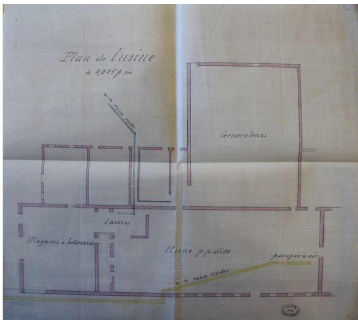
Plan détaillé de la sucrerie de Berneuil-sur-Aisne, 1893. (AD Oise ; Mp 2421).
