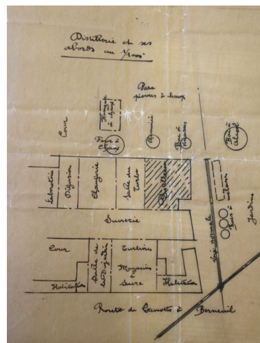
Plan masse de situation pour l'implantation de la nouvelle distillerie de la sucrerie, 1936 (AD Oise ; Mp 2421). Phot. Bertrand Fournier IVR22_20116001034NUCAB
