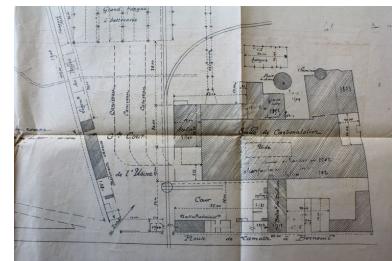
Plan masse de la sucrerie, avec indication des dates de construction des bâtiments, 1932 (AD Oise ; 10 Rp 1865). Phot. Bertrand Fournier IVR22_20116001032NUCAB
