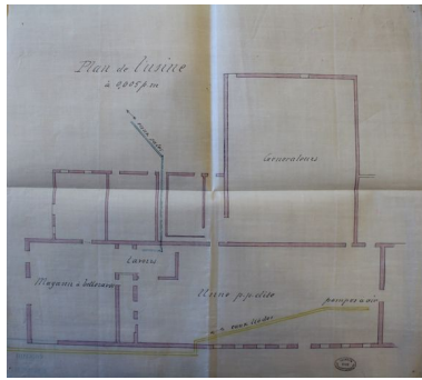
Plan détaillé de la sucrerie de Berneuil-sur-Aisne, 1893. (AD Oise ; Mp 2421). Phot. Bertrand Fournier IVR22_20106001024NUCA
