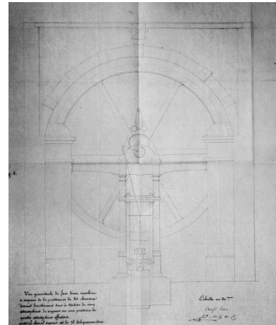
Vue générale de face d'une machine à vapeur de la puissance de 20 chevaux, échelle 1/20e, 1852 (AD Oise ; 5M). Phot. Benoît Dufournier IVR22_19936001602ZB
