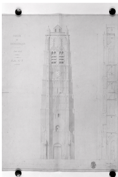
Tour : coupe partielle, élévation de la façade est. Phot. Jean-Michel Périn IVR31_19875903370X
