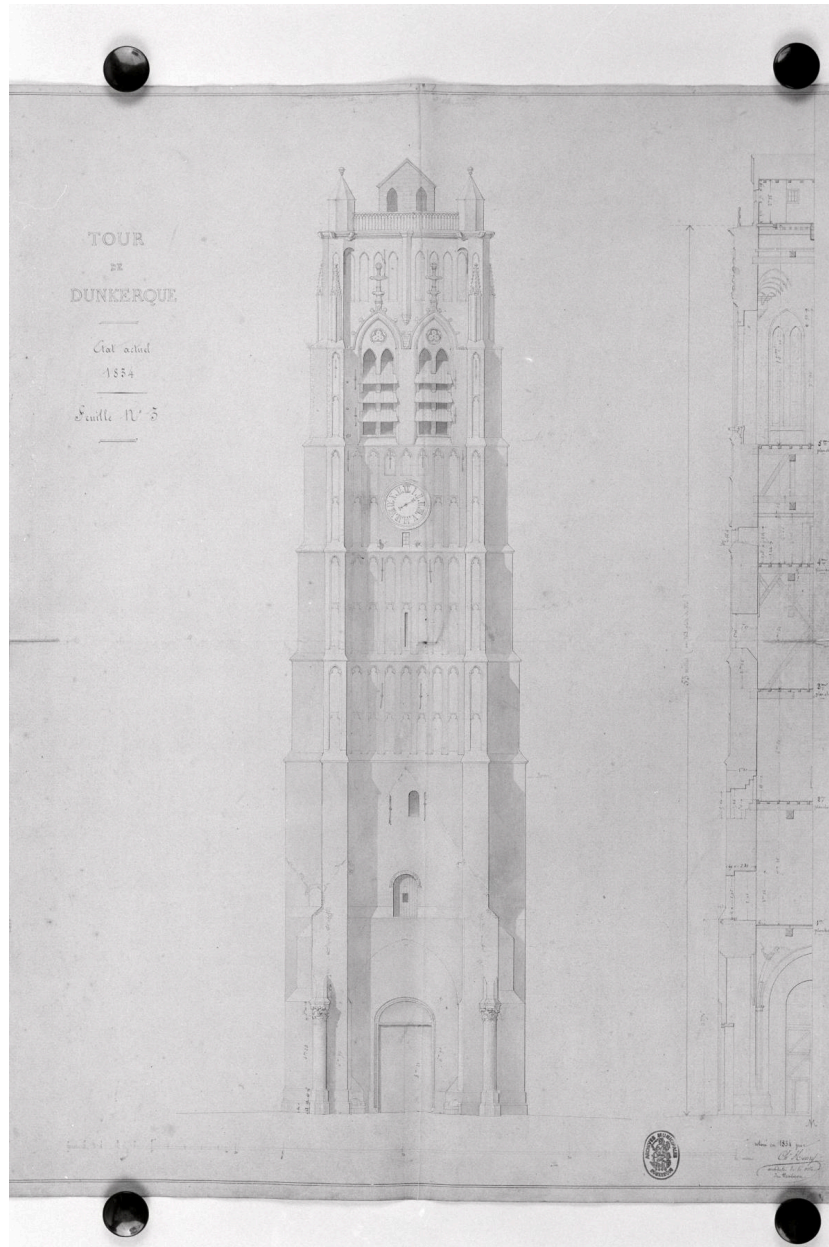
Tour : coupe partielle, élévation de la façade est.
