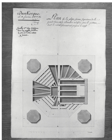
Plan de la plate-forme supérieure de la grande tour et de la chambre au-dessus pour le guetteur dont le rétablissement est proposé à neuf.
