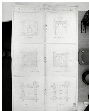
Tour, plans : 4e et 5e niveaux, plancher haut de la chambre des cloches, charpente portant la plate-forme, plate-forme, Tour, coupes : dernier niveau, loge du guetteur.
