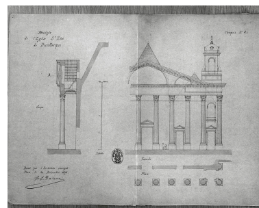
Plan partiel et coupe du péristyle, élévation partielle de la façade. Phot. Jean-Michel Périn IVR31_19875902943X
