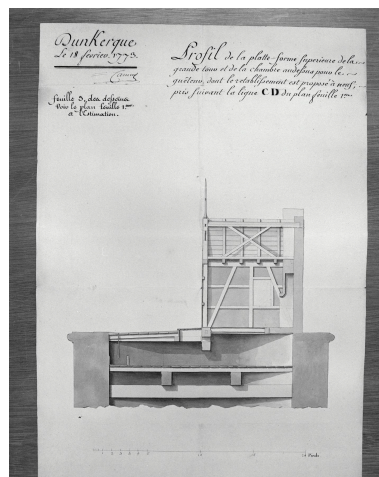
Profil de la plate-forme supérieure de la grande tour et de la chambre au-dessus pour le guetteur, dont le rétablissement est proposé à neuf, pris suivant la ligne CD du plan feuille 1ère.
