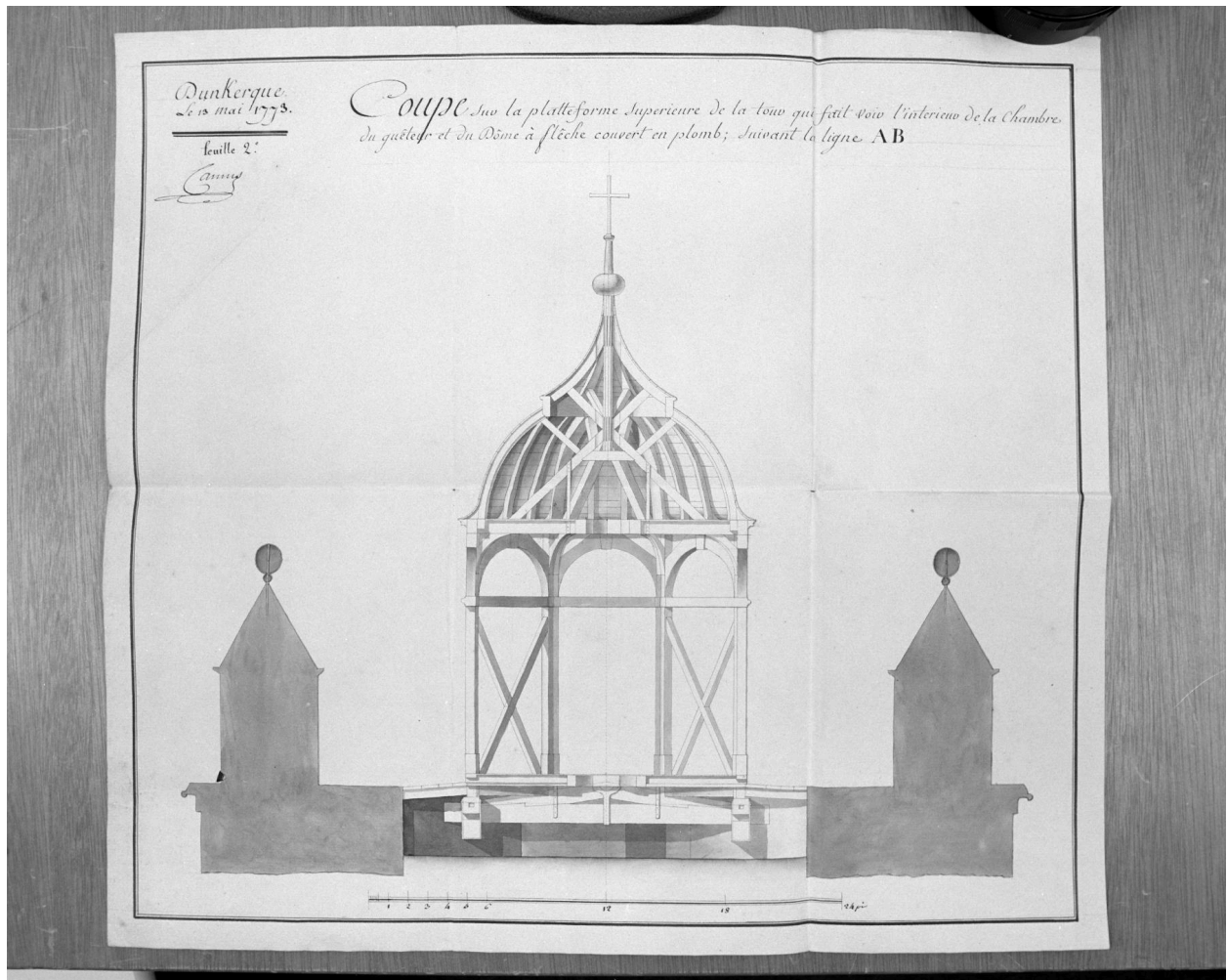
Coupe sur la plate-forme supérieure de la tour, coupe du belvédère, projet.
