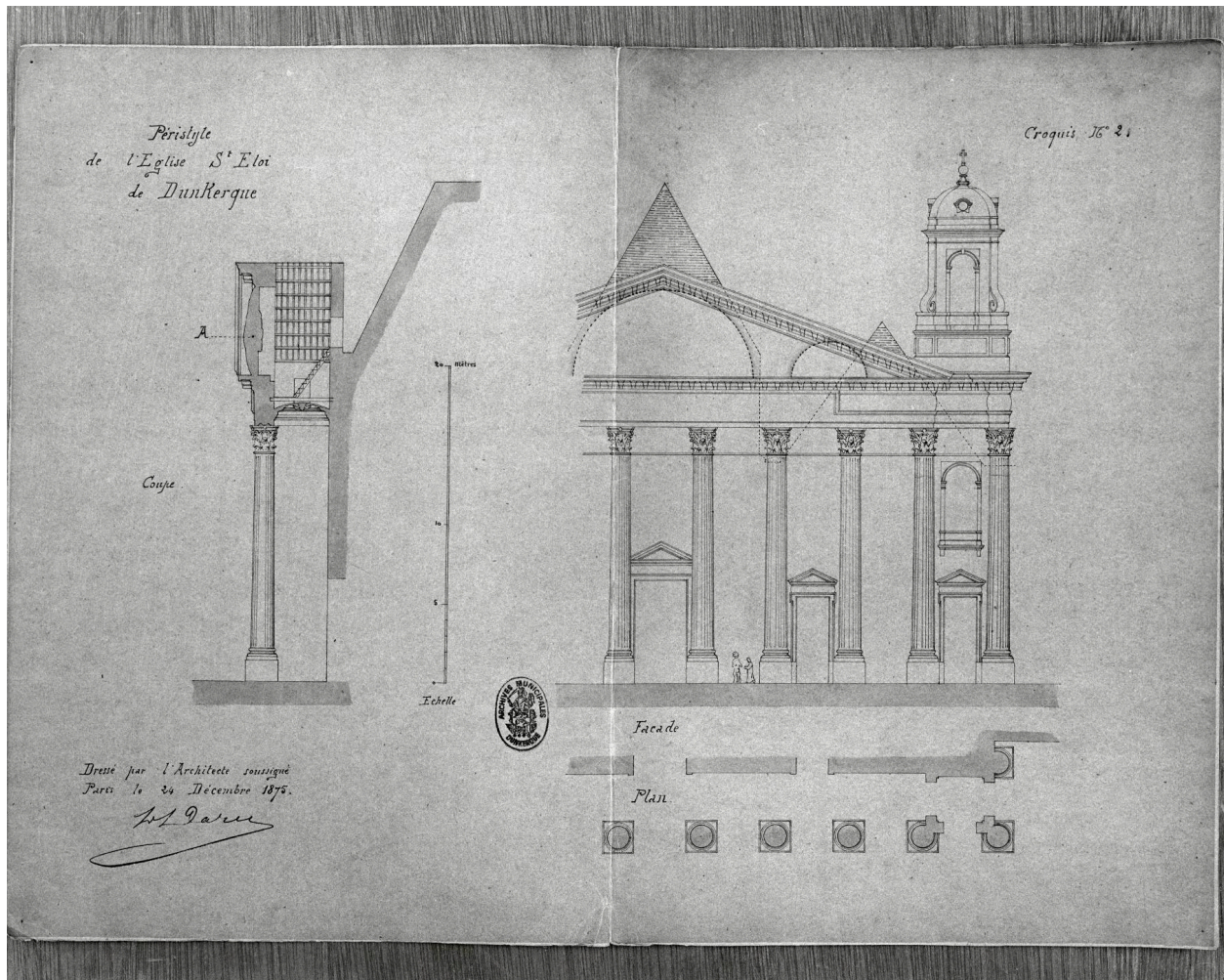
Plan partiel et coupe du péristyle
