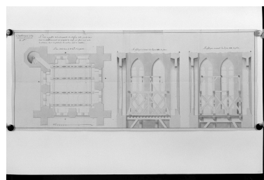
Plan et profils de la charpente du beffroi de la grande tour dont le rétablissement est proposé à neuf, qui font aussi voir les vitraux dont les piédroits du milieu sont à rétablir. Phot. Jean-Michel Périn IVR31_19875903457X
