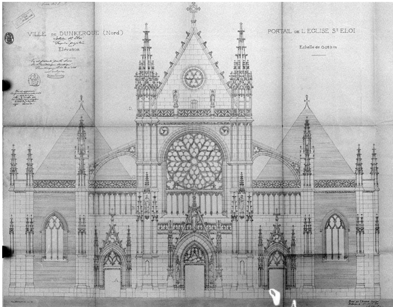
Projet de reconstruction de la façade, élévation.
