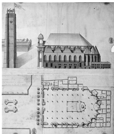
Plan, élévation des façades latérales de l'église et de la tour, après les transformations apportées par V. Louis, après 1785.
