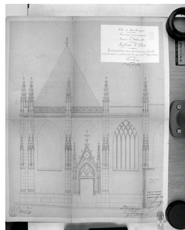
Projet de rhabillage du début de la façade latérale sud, élévation. Phot. Jean-Michel Périn IVR31_19875902936X
