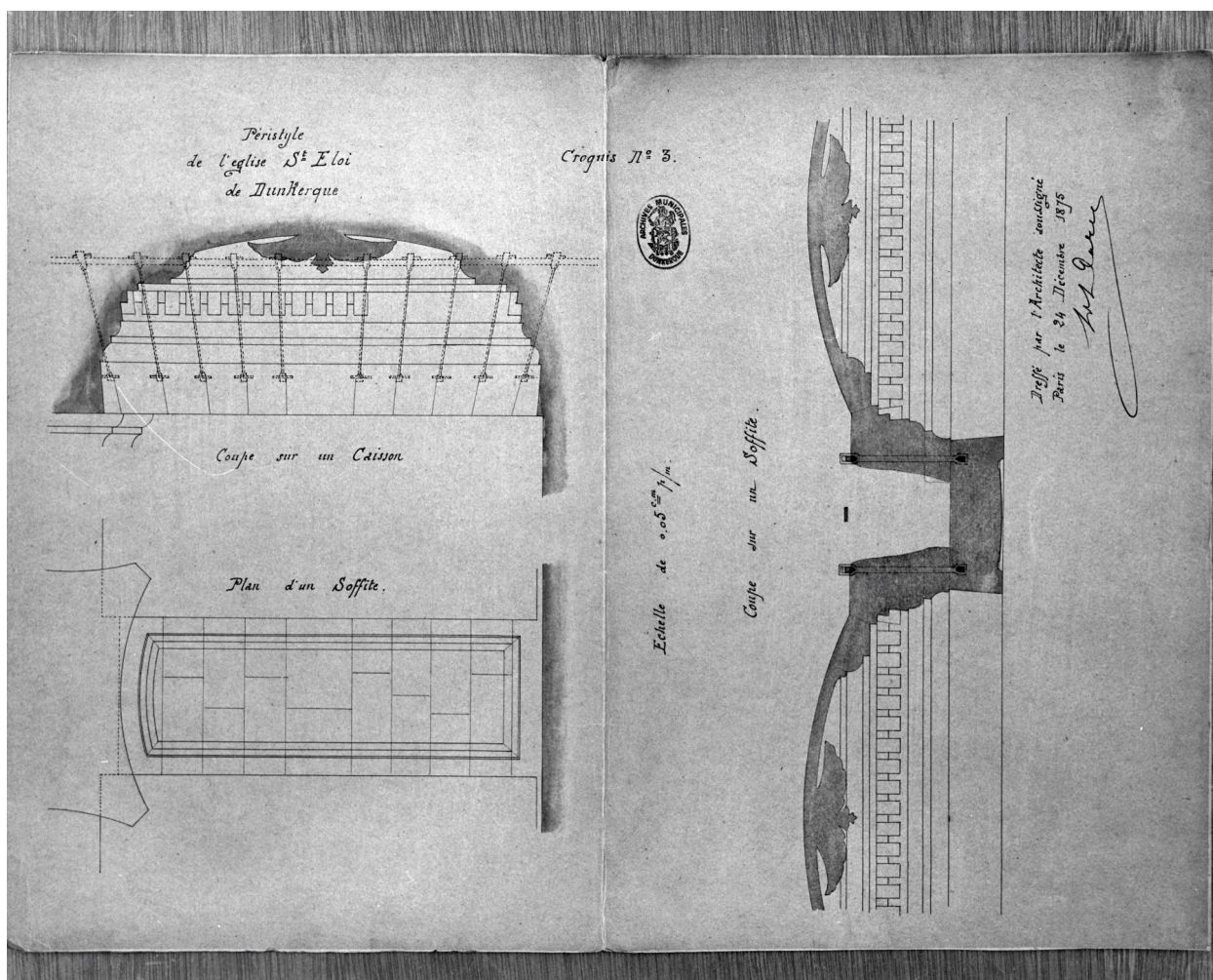
Péristyle, détails : coupe et plan d'un soffite, coupe sur un caisson.
