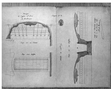
Péristyle, détails : coupe et plan d'un soffite, coupe sur un caisson. Phot. Jean-Michel Périn IVR31_19875902942X
