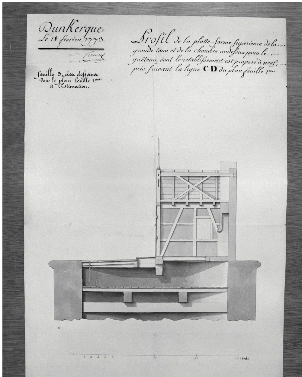
Profil de la plate-forme supérieure de la grande tour et de la chambre au-dessus pour le guetteur, dont le rétablissement est proposé à neuf, pris suivant la ligne CD du plan feuille 1ère.
