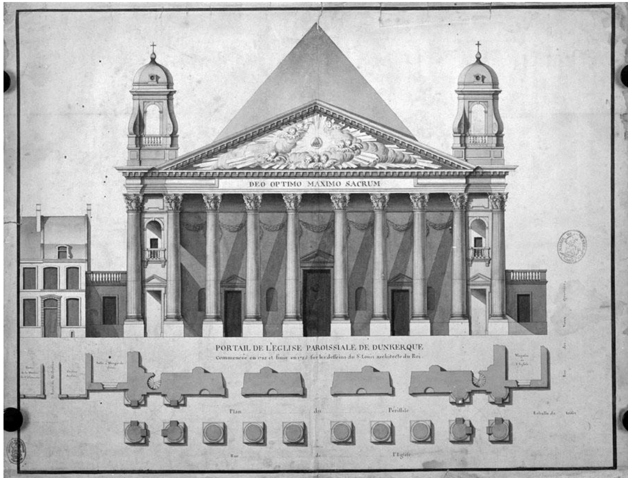
Plan du péristyle et du mur de façade de l'église, élévation de la façade principale de l'église et de la façade du presbytère, vers 1785.
