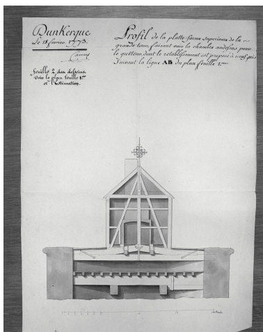
Profil de la plate-forme supérieure de la grande tour faisant voir la chambre au-dessus pour le guetteur, dont le rétablissement est proposé à neuf, pris suivant la ligne AB du plan feuille 1ère.
