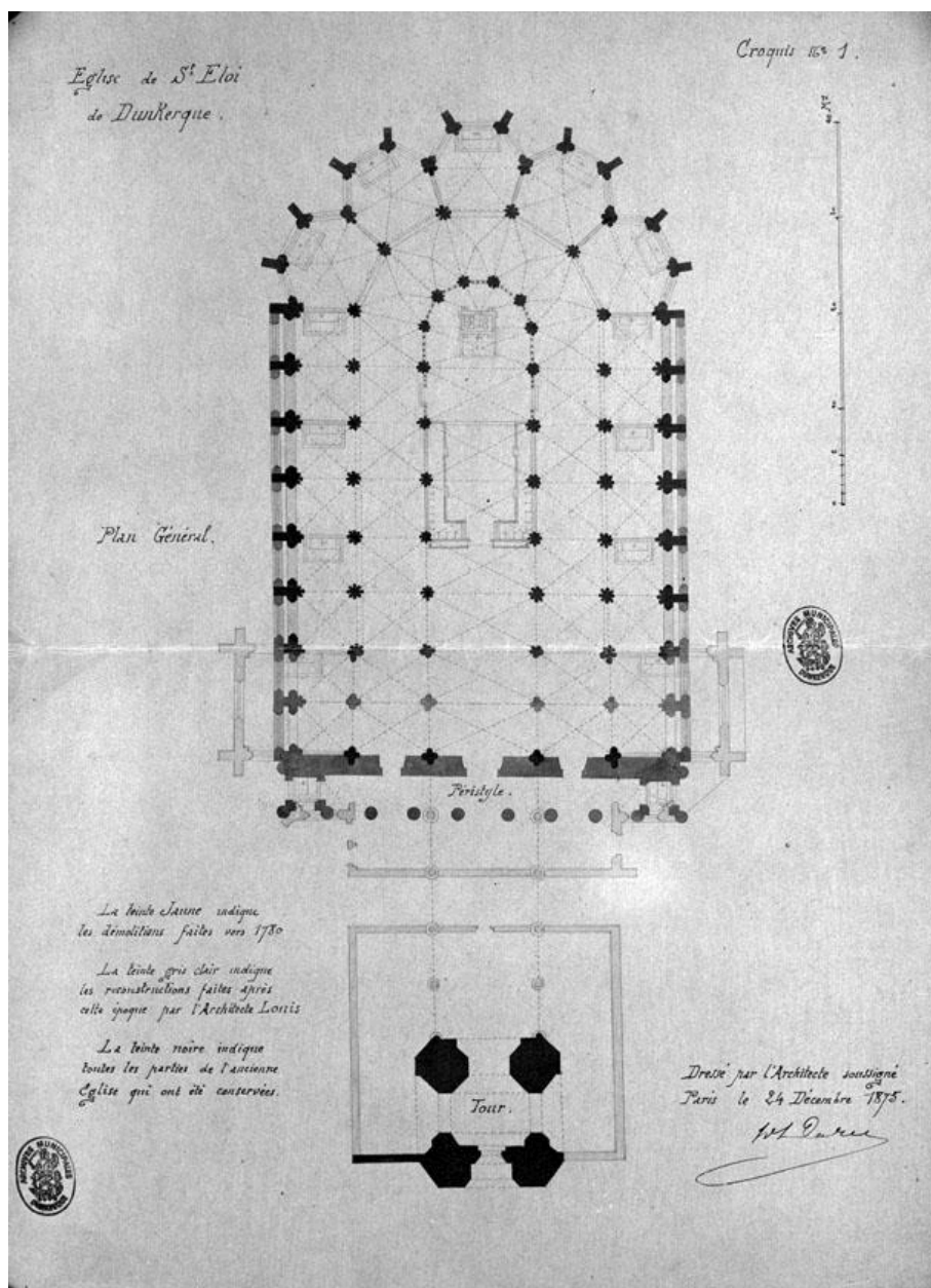
Plan de l'église et de la tour.
