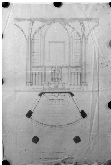
Plan et élévation de la chapelle du Saint-Sacrement dans son état actuel. Phot. Jean-Michel Périn IVR31_19885902001X
