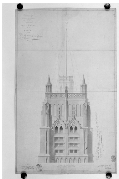
Tour : projet de restauration de la partie supérieure. Phot. Jean-Michel Périn IVR31_19875903371X
