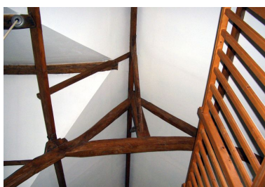
Vue de la charpente de l'ancienne grange. Phot. Inès Guérin IVR22_20058005092NUCA
