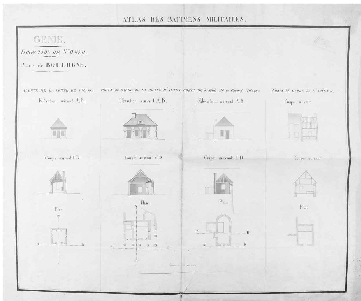
Plan, coupe, façade. Atlas des bâtiments militaires, génie, direction Saint Omer. Archives privées.
