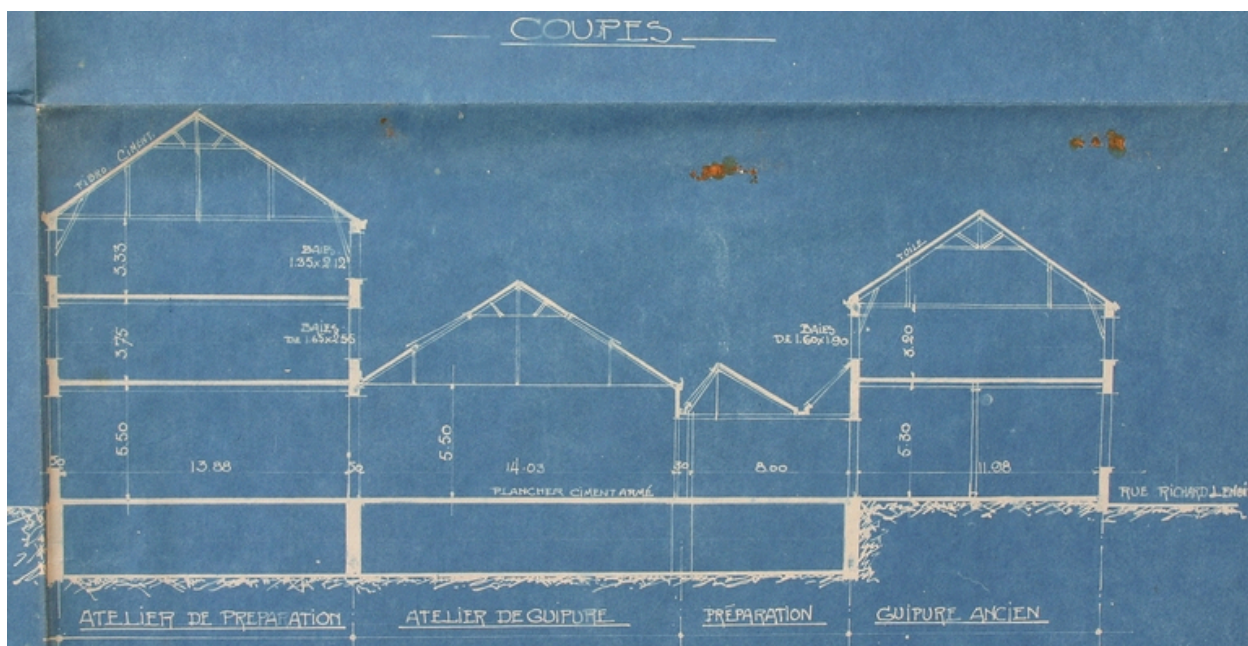
Coupe transversale des ateliers vers 1920 (AD Aisne).
