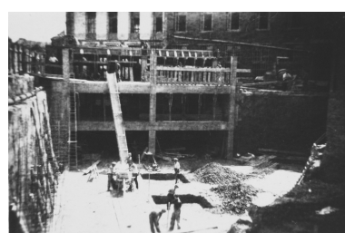
Construction des fondations des ateliers à l'angle des rues Camille-Desmoulins et de Mulhouse, 1947 (IFA). Phot. Pillet Frédéric IVR22_20040201140NUCAB
