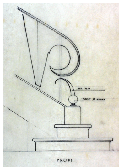
Plan de détail du départ de la rampe d'escalier, par Denis Honegger, 1949 (IFA). Phot. Pillet Frédéric IVR22_20040201137NUCAB
