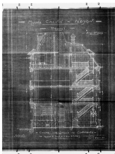
Coupe sur la salle de conférence. Projet de restauration, par Letrosne, 1927 (AC Noyon). Repro. Monnehay- Vulliet Marie-Laure IVR22_20096000516NUCA
