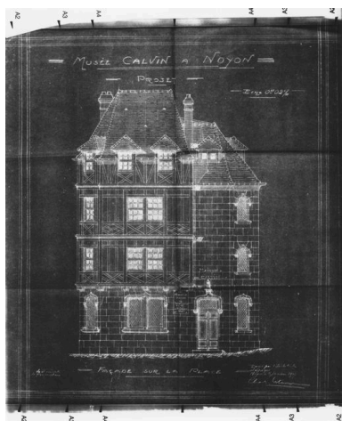
Elévation antérieure. Projet de restauration, par Letrosne, 1927 (AC Noyon). Repro. Monnehay- Vulliet Marie-Laure IVR22_20096000517NUCA
