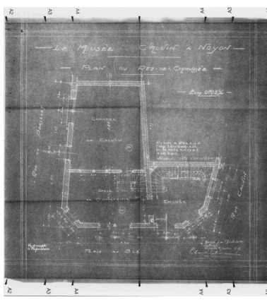
Plan au sol. Projet de restauration, par Letrosne, 1927 (AC Noyon). Repro. Monnehay-Vulliet Marie-Laure IVR22_20096000514NUCA
