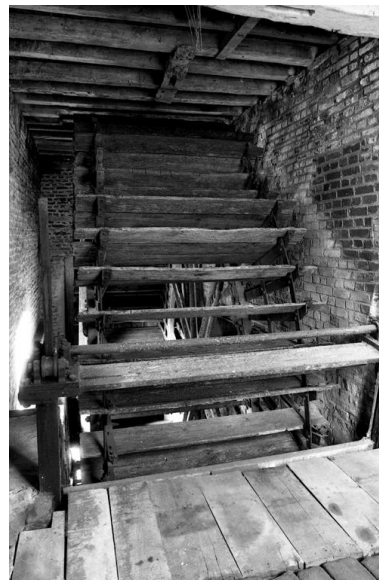
Vue de la roue hydraulique verticale, à l'arrêt. Phot. Thierry Lefébure IVR22_19920201201Z
