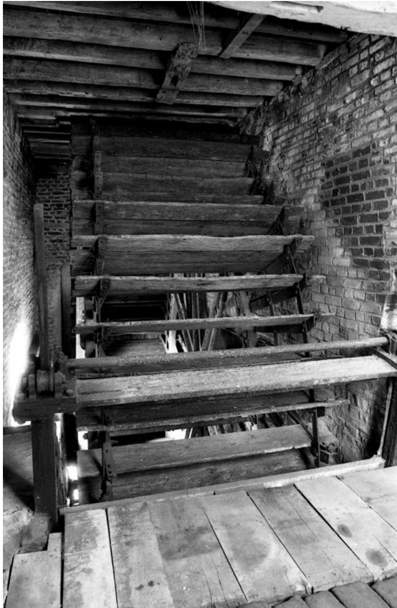
Vue de la roue hydraulique verticale, à l'arrêt.
