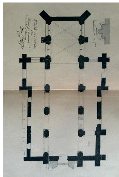
Plan au sol. Phot. Bertrand Fournier IVR22_20138015849NUC2A
