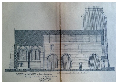
Coupe longitudinale. Phot. Bertrand Fournier IVR22_20138015850NUC2AQ
