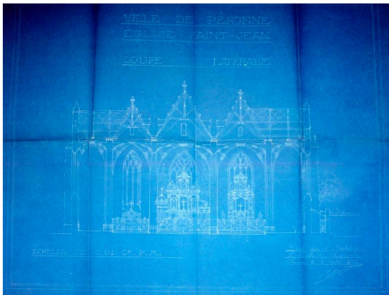
Coupe latérale, Daniel Roguet (architecte), 5 juillet 1921 (AD Somme ; 10 R 1032).
