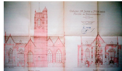
Projet de restauration d'après l'état d'avant guerre, façades nord et ouest, Henry Moreau (architecte en chef des Monuments Historiques), août 1924 (AD Somme ; 99 O 3000). Phot. Gilles-Henri Bailly IVR22_20158005609NUCA
