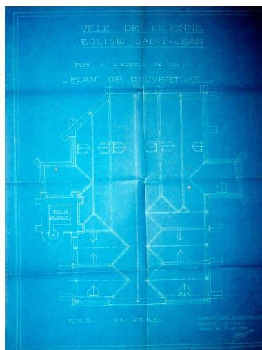
Plan de la couverture, Daniel Roguet (architecte), 3 mars 1921 (AD Somme ; 10 R 1032). Phot. Gilles-Henri Bailly IVR22_20158005614NUCA
