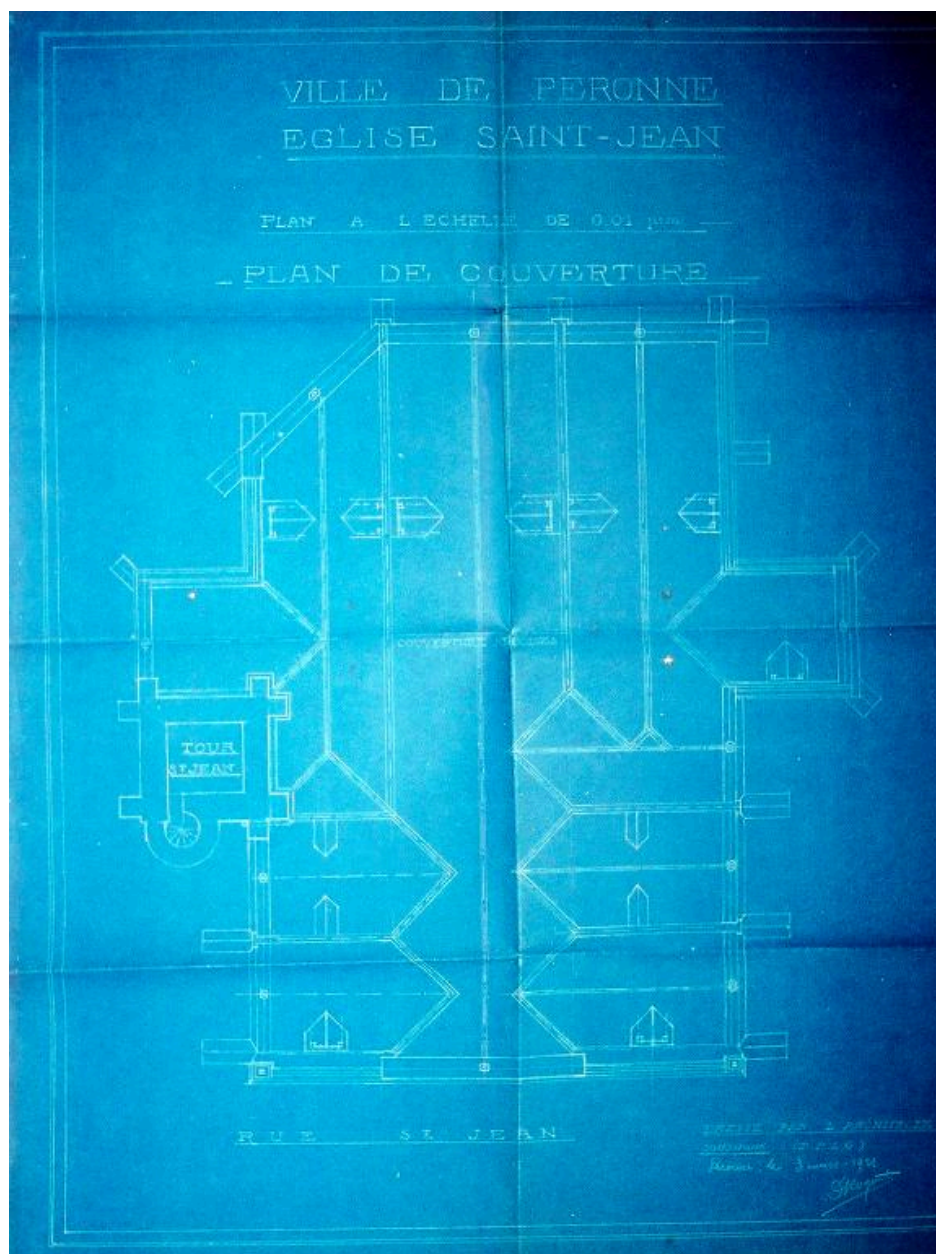
Plan de la couverture, Daniel Roguet (architecte), 3 mars 1921 (AD Somme ; 10 R 1032).
