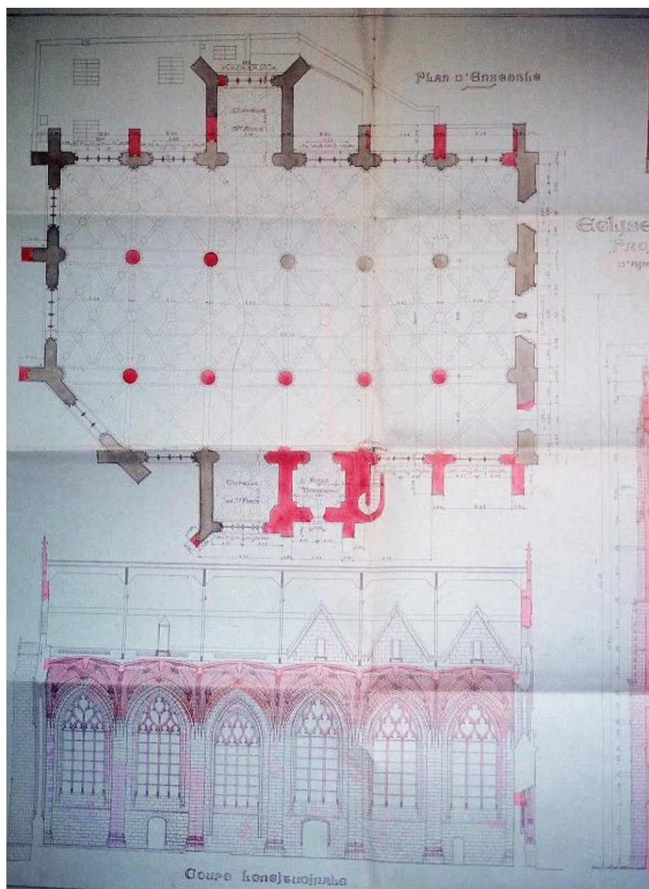
Projet de restauration d'après l'état d'avant guerre, plan d'ensemble, coupe longitudinale, Henry Moreau (architecte en chef des Monuments Historiques), 31 janvier 1925 (AD Somme ; 10 R 1032).
