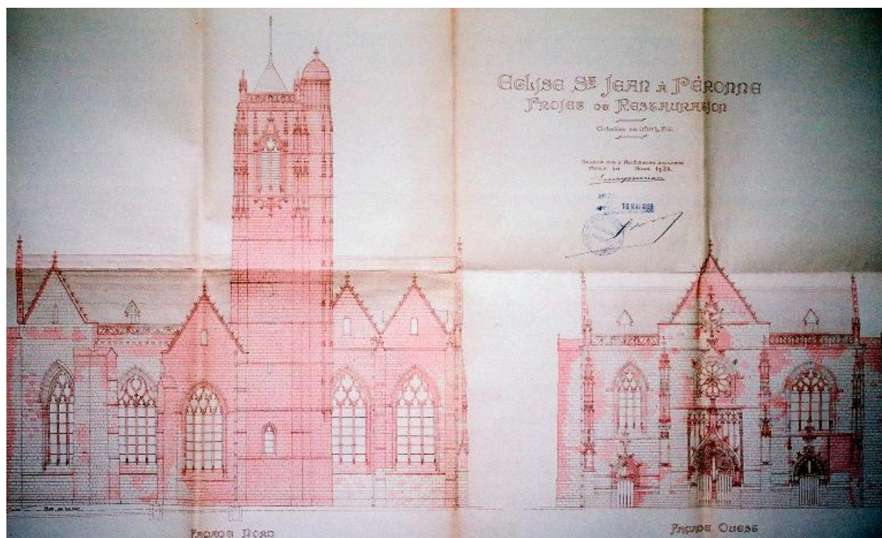
Projet de restauration d'après l'état d'avant guerre, façades nord et ouest, Henry Moreau (architecte en chef des Monuments Historiques), août 1924 (AD Somme ; 99 O 3000).
