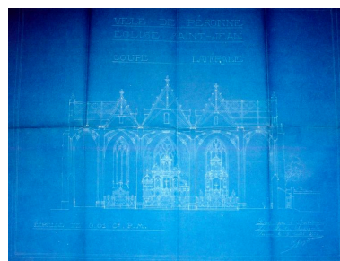
Coupe latérale, Daniel Roguet (architecte), 5 juillet 1921 (AD Somme ; 10 R 1032). Phot. Gilles-Henri Bailly IVR22_20158005615NUCA
