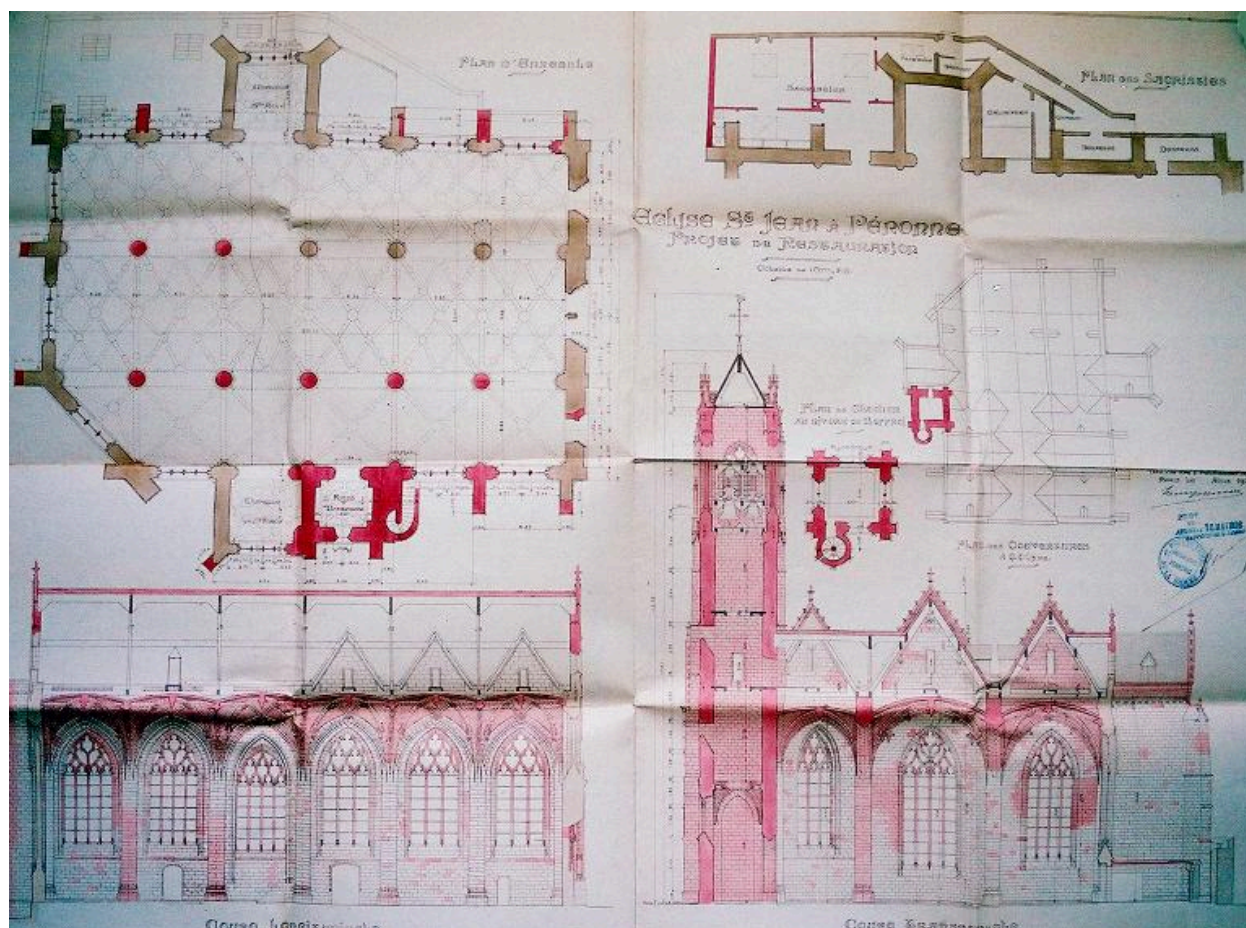
Projet de restauration d'après l'état d'avant guerre, plan d'ensemble, plan des sacristies, plan du clocher, Henry Moreau (architecte en chef des Monuments Historiques), août 1924 (AD Somme ; 99 O 3000).
