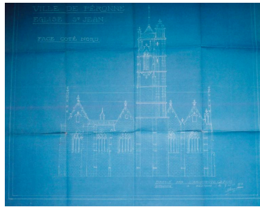
Façade côté nord, Daniel Roguet (architecte), 7 avril 1921 (AD Somme ; 10 R 1032). Phot. Gilles-Henri Bailly IVR22_20158005617NUCA
