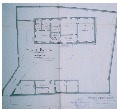
Plan du presbytère, Coulombel (architecte conducteur des travaux de la ville), 15 novembre 1920 (AD Somme ; 10 R 1032). Phot. Gilles-Henri Bailly IVR22_20158005618NUCA
