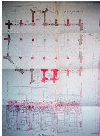
Projet de restauration d'après l'état d'avant guerre, plan d'ensemble, coupe longitudinale, Henry Moreau (architecte en chef des Monuments Historiques), 31 janvier 1925 (AD Somme ; 10 R 1032). Phot. Gilles-Henri Bailly IVR22_20158005607NUCA
