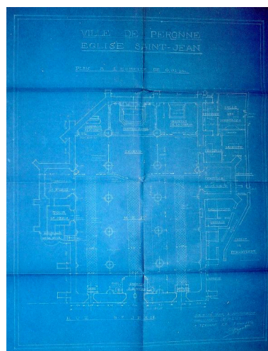
Plan de l'église, Daniel Roguet (architecte), 3 mars 1921 (AD Somme ; 10 R 1032). Phot. Gilles-Henri Bailly IVR22_20158005612NUCA
