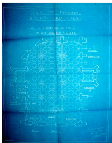
Plan de la voûte, Daniel Roguet (architecte), 3 mars 1921 (AD Somme ; 10 R 1032). Phot. Gilles-Henri Bailly IVR22_20158005613NUCA
