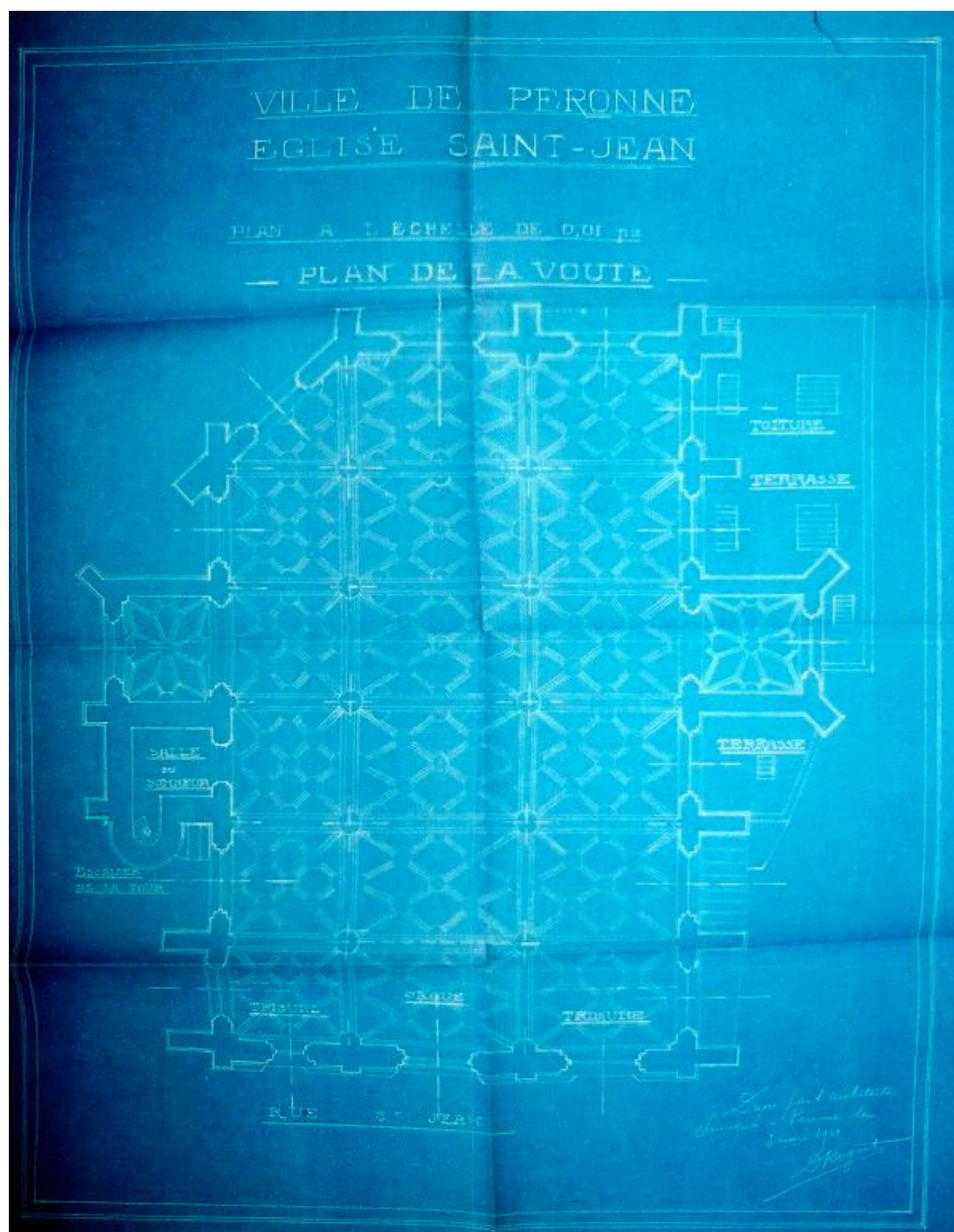
Plan de la voûte, Daniel Roguet (architecte), 3 mars 1921 (AD Somme ; 10 R 1032).
