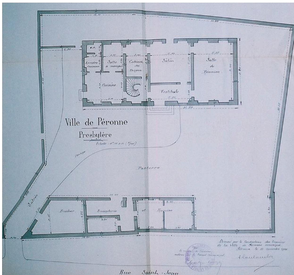
Plan du presbytère, Coulombel (architecte conducteur des travaux de la ville), 15 novembre 1920 (AD Somme ; 10 R 1032).
