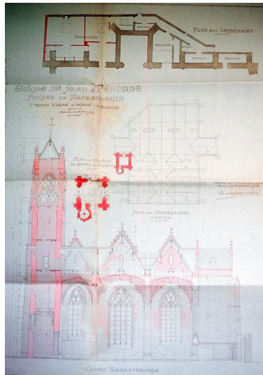
Projet de restauration d'après l'état d'avant guerre, plan des sacristies et plan du clocher, Henry Moreau (architecte en chef des Monuments Historiques), 31 janvier 1925 (AD Somme ; 10 R 1032). Autre exemplaire, août 1924 (AD Somme ; 99 O 3000). Phot. Gilles-Henri Bailly IVR22_20158005608NUCA
