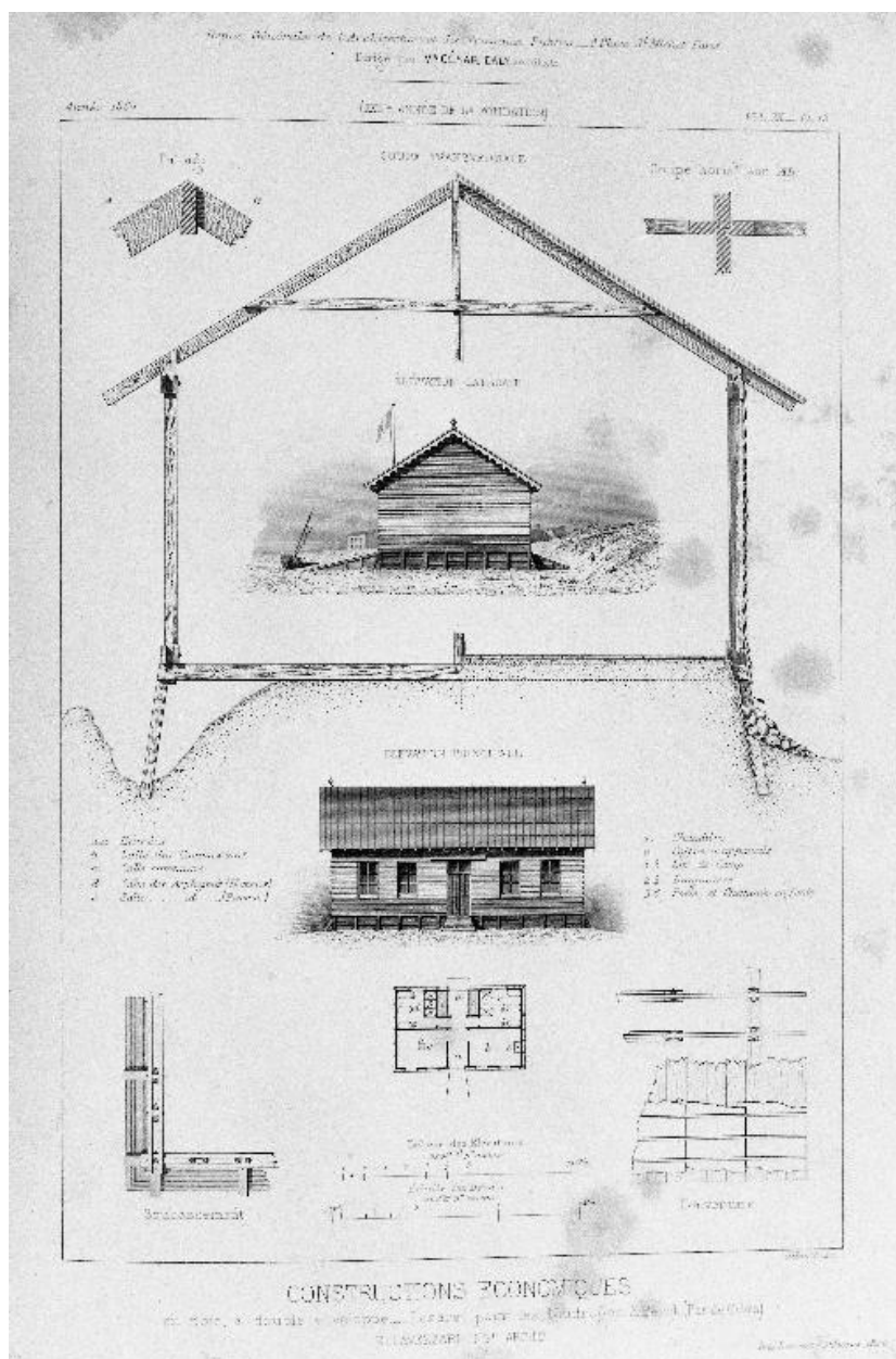
Planche illustrant le mode de construction de l'édifice baptisé ultérieurement petit hôpital maritime bien que les deux élévations visibles montrent un autre exemple d'édifice relevant du même mode de construction. Extrait de Revue générale de l'architecture et des travaux publics, tome XX, 1862, pl. 13.
