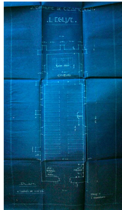
Plan de l'église détruite, par Jean Antoine (architecte), [s.d.] (AD Somme ; 10 R 331). Phot. Gilles-Henri Bailly (reproduction) IVR22_20158005441NUCA
