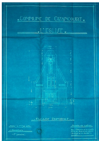
Façade principale, projet de reconstruction par Jean Antoine (architecte), 1er mai 1926 (AD Somme ; 99 O 1171). Phot. Gilles-Henri Bailly (reproduction) IVR22_20158005448NUCA
