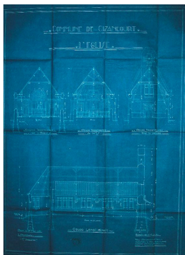
Coupes longitudinale et transversales, projet de reconstruction par Jean Antoine (architecte), 1er mai 1926 (AD Somme ; 99 O 1171). Phot. Gilles-Henri Bailly (reproduction) IVR22_20158005446NUCA
