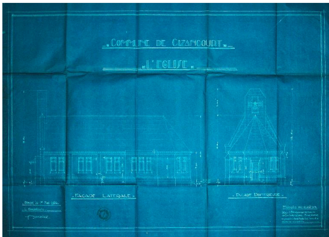
Façades latérale et postérieure, projet de reconstruction par Jean Antoine (architecte), 1er mai 1926 (AD Somme ; 99 O 1171).
