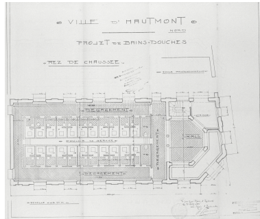
Projet de bains-douches (rez-de-chaussée) dressé par la Société de Bains-Douches, Lavoires et Travaux municipaux, Paris, Léon Perreau architecte, 1912 (non réalisé) (AD Nord ; série O 285/176). Repro. Olivier Marlard IVR31_19925901256X
