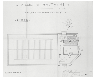
Projet de bains-douches (étage) dressé par la Société de Bains-Douches, Lavoires et Travaux municipaux, Paris, Léon Perreau architecte, 1912 (non réalisé) (AD Nord ; série O 285/176). Repro. Olivier Marlard IVR31_19925901255X
