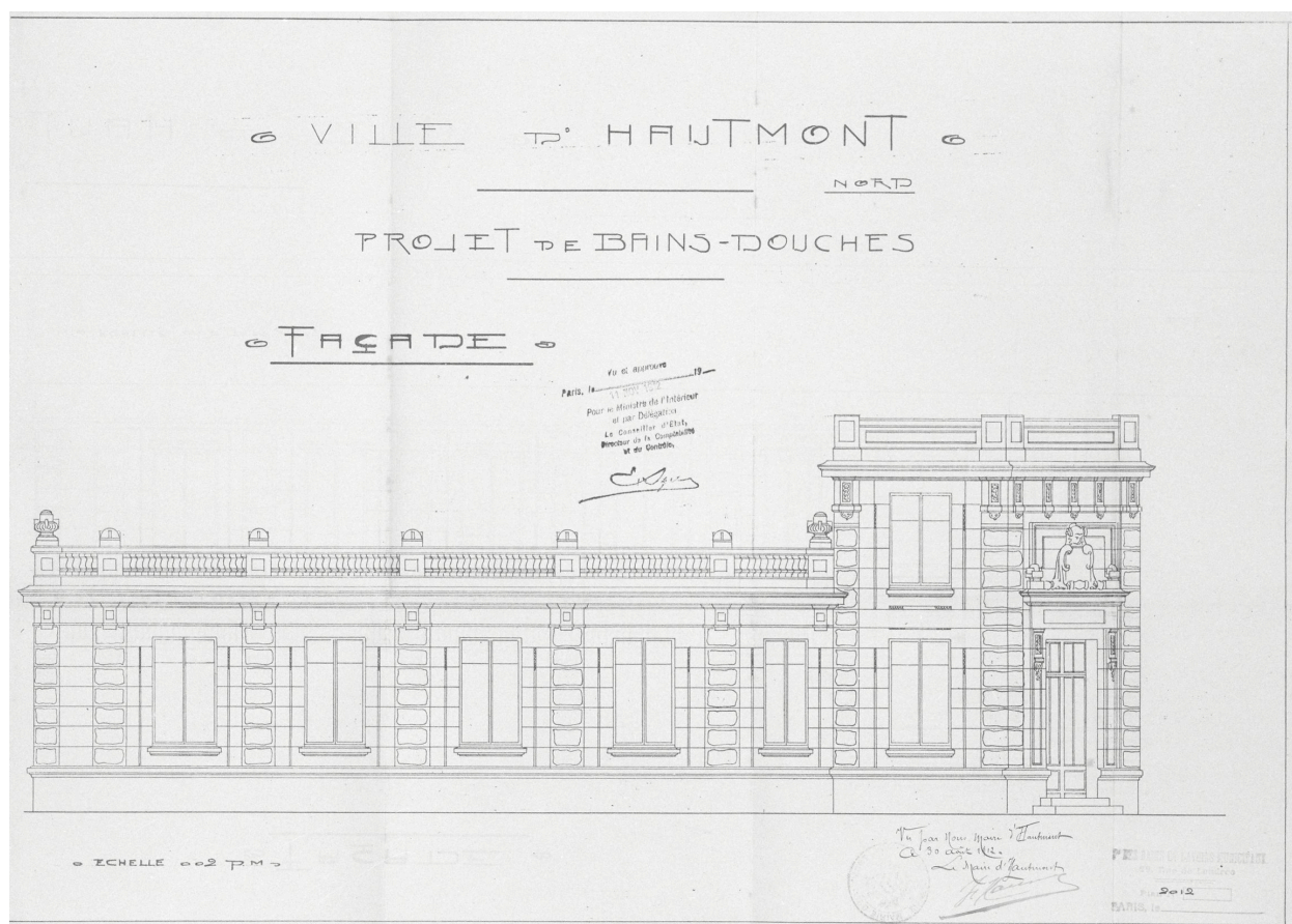
Projet de bains-douches (façade) dressé par la Société de Bains-Douches, Lavoires et Travaux municipaux, Paris, Léon Perreau architecte, 1912 (non réalisé) (AD Nord ; série O 285/176).
