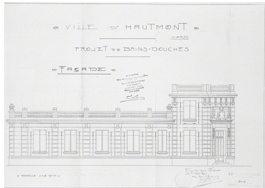
Projet de bains-douches (façade) dressé par la Société de Bains-Douches, Lavoires et Travaux municipaux, Paris, Léon Perreau architecte, 1912 (non réalisé) (AD Nord ; série O 285/176). Repro. Olivier Marlard IVR31_19925901254X
