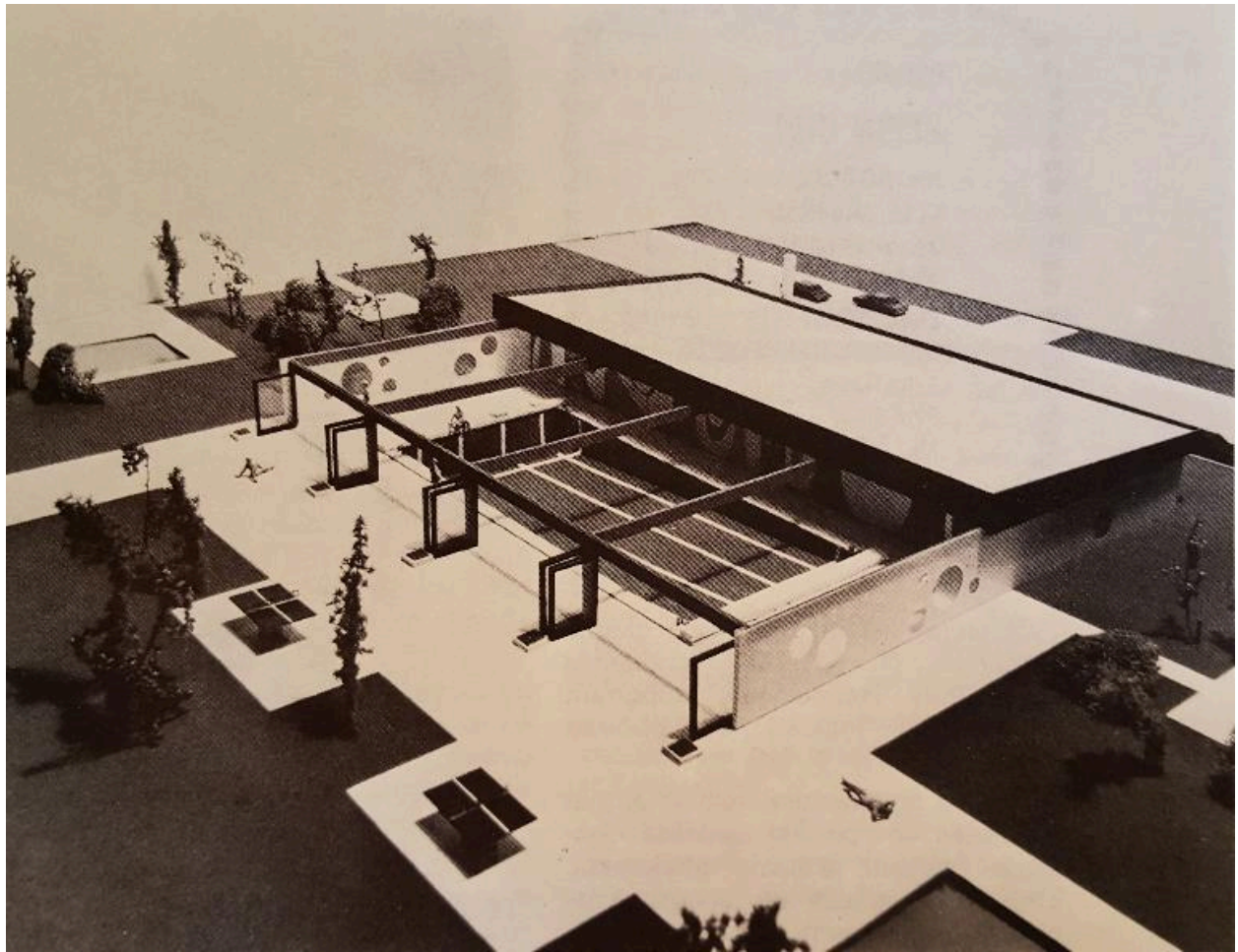
Maquette de la piscine Plein Soleil, photographie. In Piscines, avril-mai 1972, n°31, p. 97.
