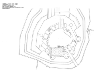
Plan du château, état en 1231, d'après copie de plan. Repro. Eddy Stein, Phot. Eddy Stein IVR31_20146202396NUC
