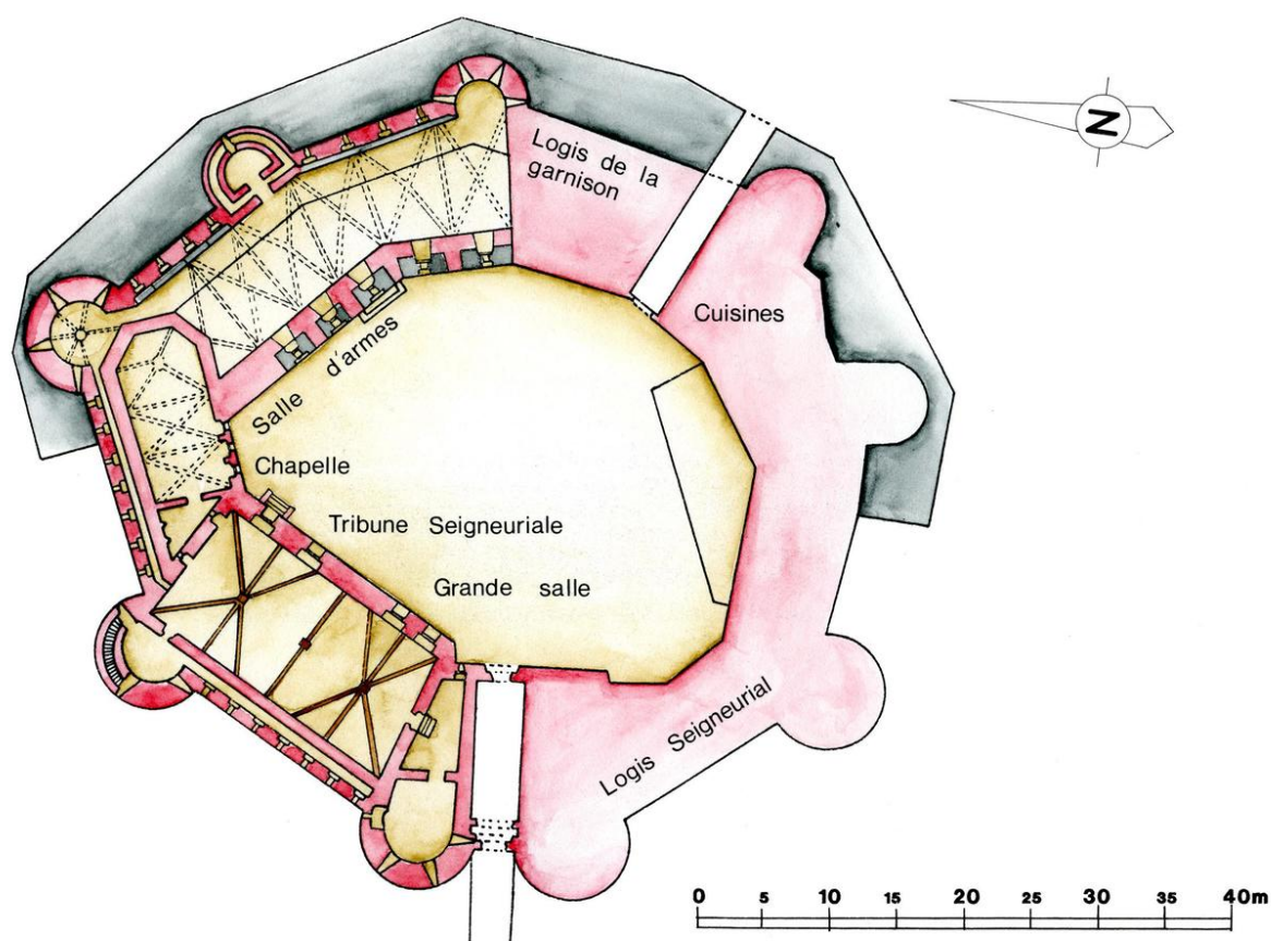
Plan restitué par Camille Enlart
