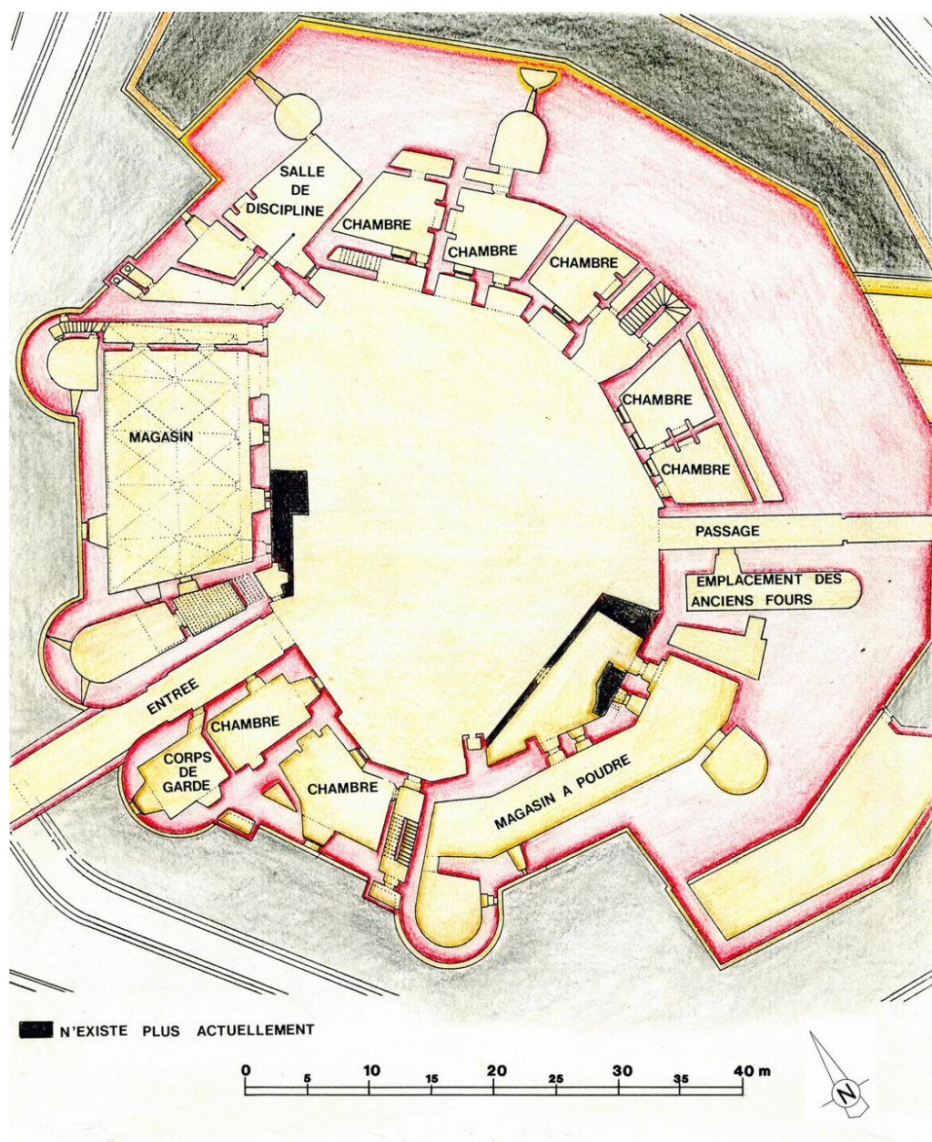
Plan du premier étage.
