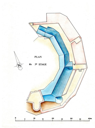
Plan du troisième étage. Repro. Eddy Stein, Phot. Eddy Stein IVR31_20116200121NUC2
