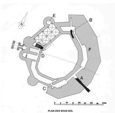
Plan du sous-sol. Repro. Eddy Stein, Phot. Eddy Stein, Phot. Hervé Leleu IVR31_20116200120NUC2
