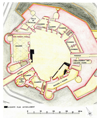
Plan du premier étage. Repro. Eddy Stein, Phot. Eddy Stein IVR31_20116200114NUC2
