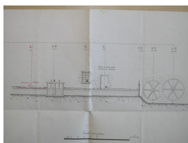
Profil annexé au rapport de l'ingénieur sur le règlement du moulin d'Hémécourt appartenant à Modeste Boileau, 26 mai 1834.
