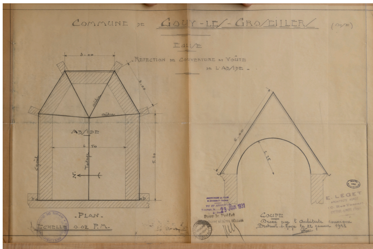
Gouy-les-Groseillers. Plan et coupe pour la réfection du chœur, 1931 (AD Oise).
