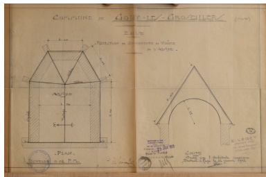
Gouy-les-Groseillers. Plan et coupe pour la réfection du chœur, 1931 (AD Oise). Repro. Marc Kérignard IVR32_20246000073NUCA
