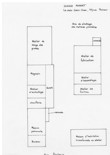
Plan schématique indiquant la fonction des bâtiments. Repro. Marie-Laure Monnehay-Vuliet, Autr. Bertrand Fournier IVR22_20106001501NUCA
