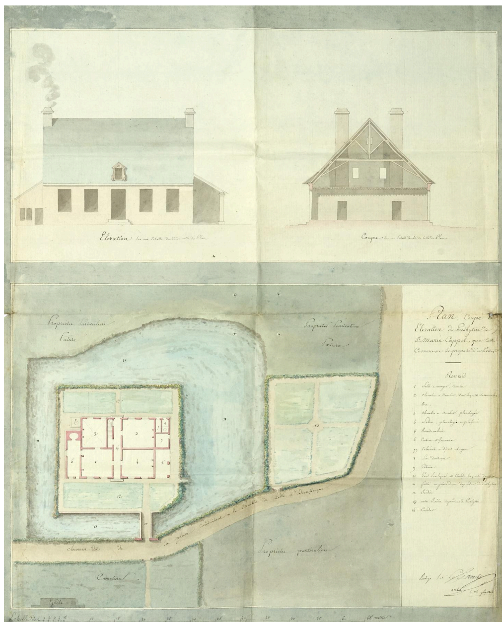
Plan, coupe, élévation du presbytère de St-Marie-Cappel, que cette commune se propose d'acheter, dressé le 25 octobre 1814 par l'architecte départemental Gesse Gervais (AD Nord : 2 O 535 / 5).
