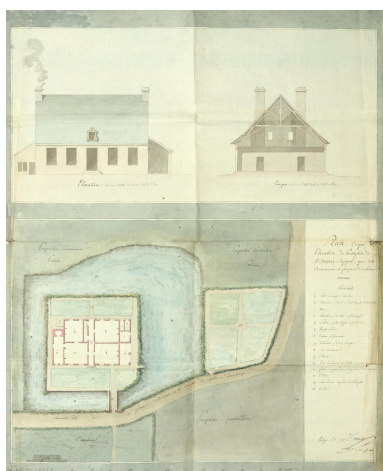
Plan, coupe, élévation du presbytère de St-Marie-Cappel, que cette commune se propose d'acheter,
