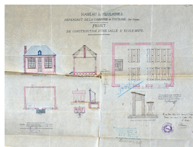
Hameau de Vieulaines. Projet de construction d'une salle d'école mixte, M. Deflesselle, architecte, 14 avril 1881 (AD Somme, 99 O 1748). Repro. Thierry Lefébure IVR32_20248000073NUCA
