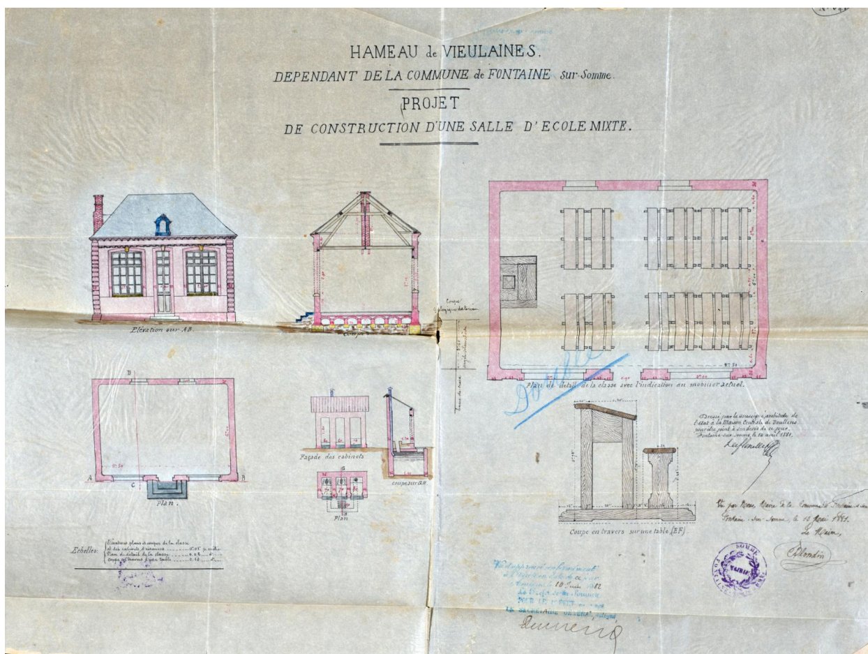
Hameau de Vieulaines. Projet de construction d'une salle d'école mixte, M. Deflesselle, architecte, 14 avril 1881 (AD Somme, 99 O 1748).
