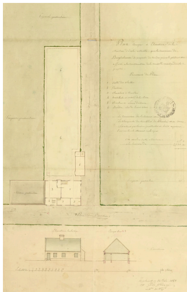
Plan, coupe et élévation de la maison d'école actuelle que la commune se propose de vendre, dressé par l'architecte départementale G. Gervais le 22 juin 1842 (AD Nord : 2 O 118/22). Repro. Delphine Volto Jourdan IVR32_20255900546NUCA
