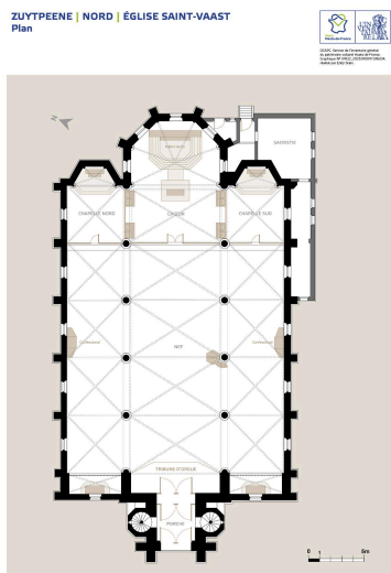
Plan de l'église. Dess. Eddy Stein IVR32_20255900915NUDA
