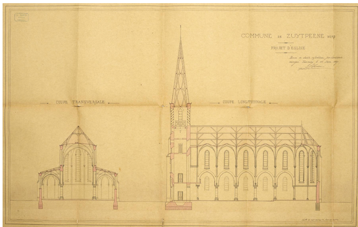
Commune de Zuytpeene, projet d'église, coupe transversale et coupe longitudinale, 1887 (AD Nord : 2 O 667 / 13).
