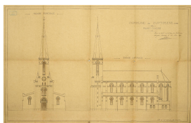
Commune de Zuytpeene, projet d'église, façade latérale, façade principale, 1887 (AD Nord : 2 O 667 / 13). Repro. Delphine Volto Jourdan IVR32_20255900053NUCA
