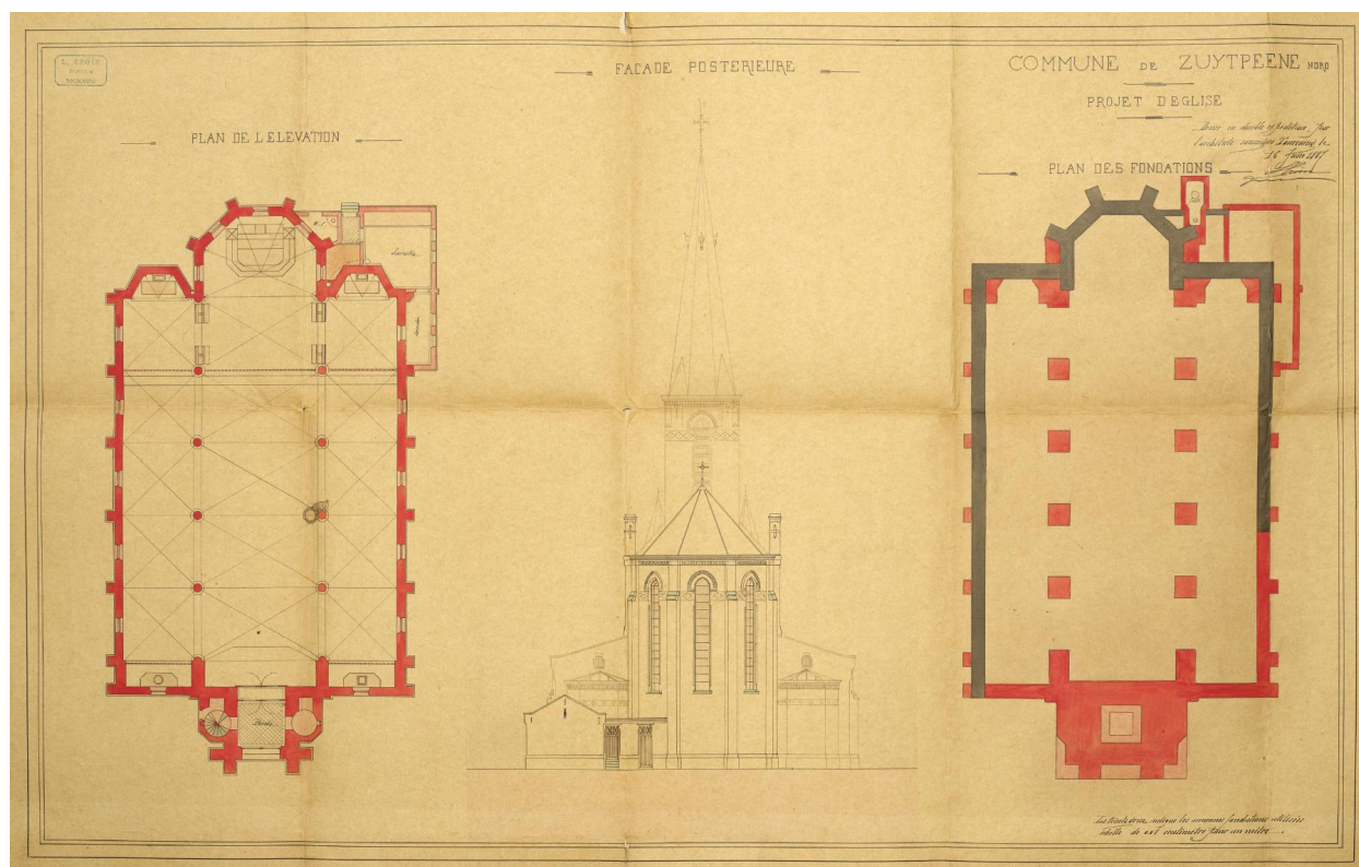
Commune de Zuytpeene, projet d'église, plan des fondations, plan de l'élévation, façade postérieure, 1887 (AD Nord : 2 O 667 / 13).
