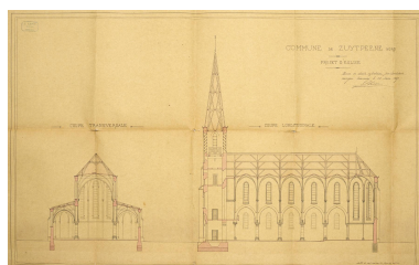
Commune de Zuytpeene, projet d'église, coupe transversale et coupe longitudinale, 1887 (AD Nord : 2 O 667 / 13). Repro. Delphine Volto Jourdan IVR32_20255900051NUCA
