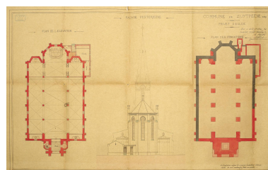
Commune de Zuytpeene, projet d'église, plan des fondations, plan de l'élévation, façade postérieure, 1887 (AD Nord : 2 O 667 / 13). Repro. Delphine Volto Jourdan IVR32_20255900052NUCA
