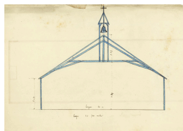
Construction d'une chapelle provisoire en remplacement de l'église incendiée, coupe, 1886 (AD Nord : 2 O 667 / 12). Repro. Delphine Volto Jourdan IVR32_20255900049NUCA
