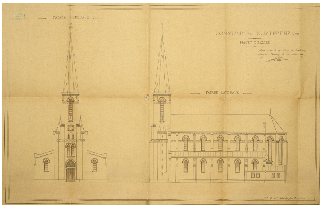
Commune de Zuytpeene, projet d'église, façade latérale, façade principale, 1887 (AD Nord : 2 O 667 / 13).
