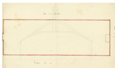
Construction d'une chapelle provisoire en remplacement de l'église incendiée, plan, 1886 (AD Nord : 2 O 667 / 12). Repro. Delphine Volto Jourdan IVR32_20255900050NUCA
