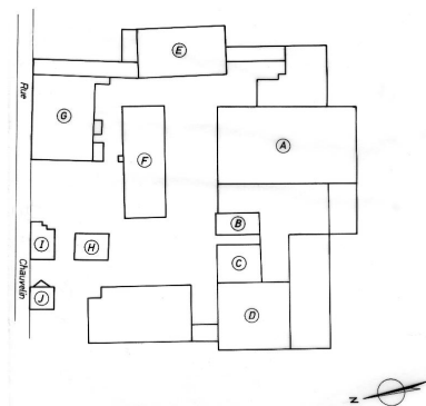
Schéma de situation : A. Ateliers de fabrication, B. Ancienne salle des machines, C. Chaufferie, D. Atelier de fabrication, E.F.G.
