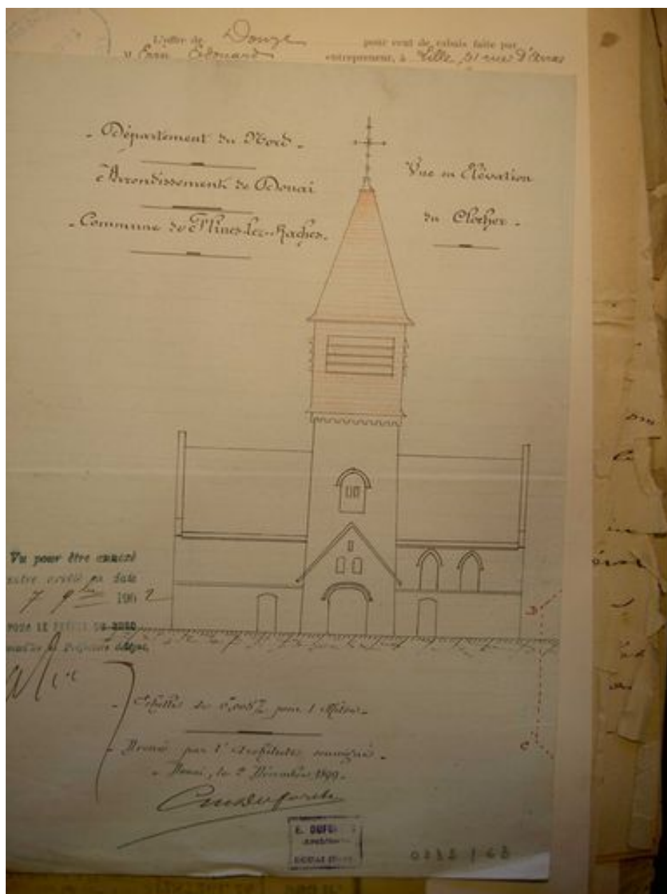
Rénovation du clocher, élévation, Emile Dufôrets architecte, 1899 (AD Nord : Série 2O 335).
