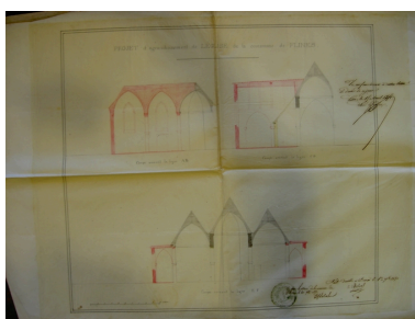
Projet d'agrandissement de l'église, coupe, Delval architecte, 1851 (AD Nord : Série 2O 335). Phot. Sophie Luchier IVR31_20075900189NUCA
