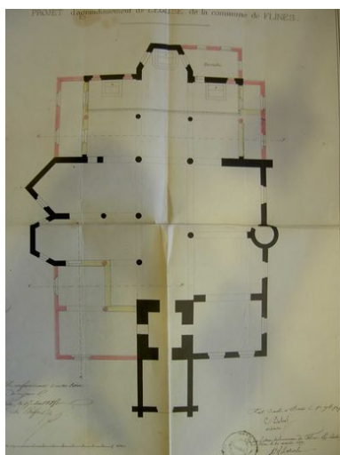
Projet d'agrandissement de l'église, plan, Delval architecte, 1851 (AD Nord : Série 2O 335). Phot. Sophie Luchier IVR31_20075900188NUCA
