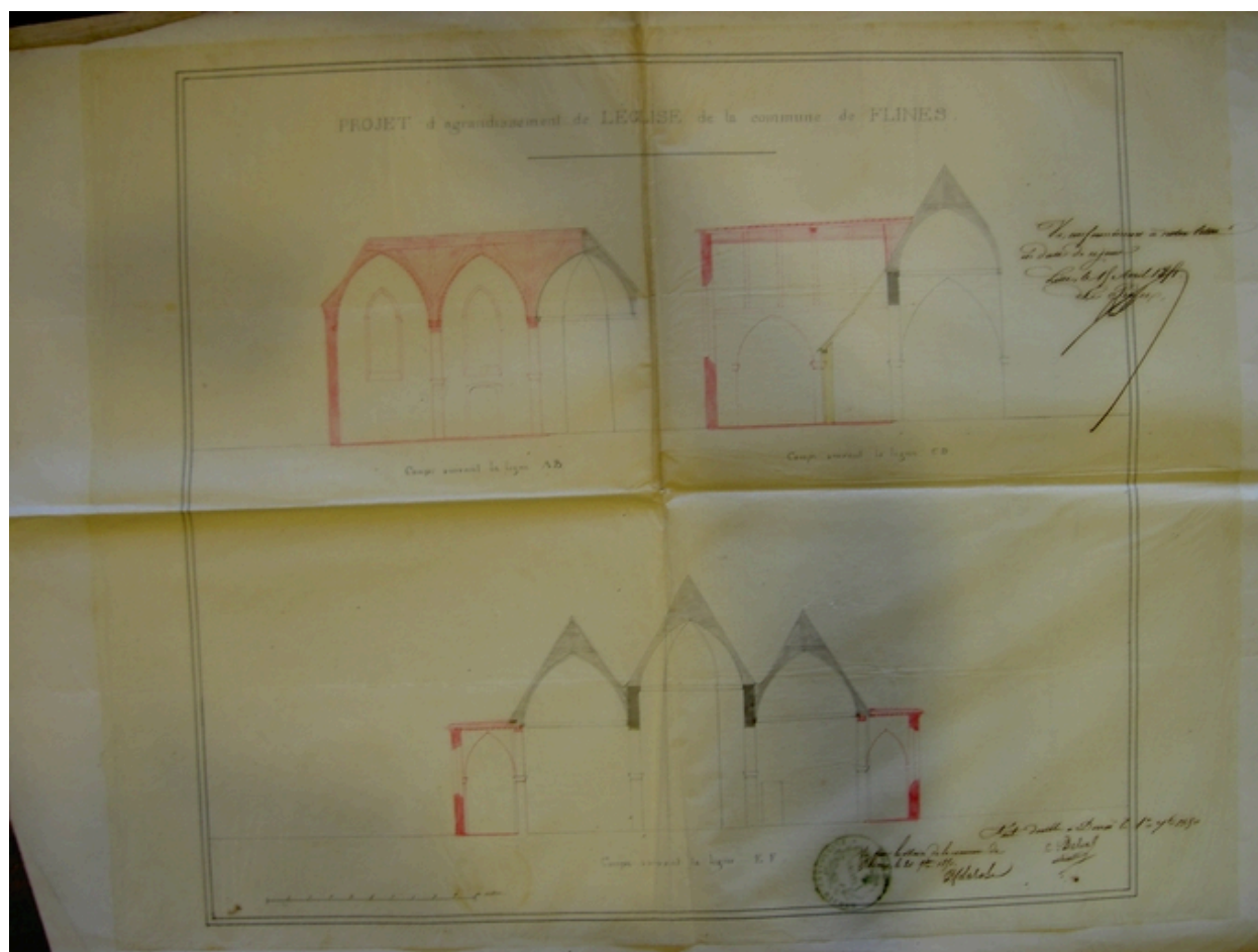
Projet d'agrandissement de l'église, coupe, Delval architecte, 1851 (AD Nord : Série 2O 335).
