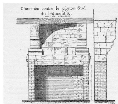
Cheminée du logis de l'ancienne ferme d'après Charles Pinsard (In : La Picardie historique et monumentale). Repro. Marie-Laure Monnehay-Vulliet IVR22_20108000045NUCA
