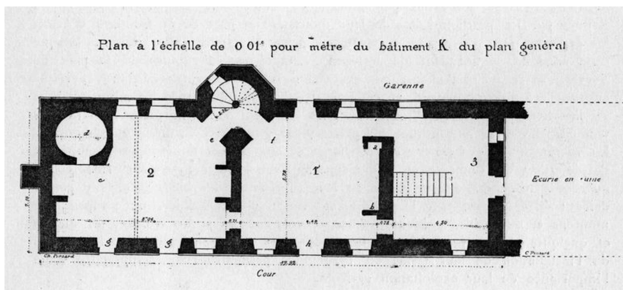
Plan de l'ancien logis d'après Charles Pinsard (In : La Picardie historique et monumentale).
