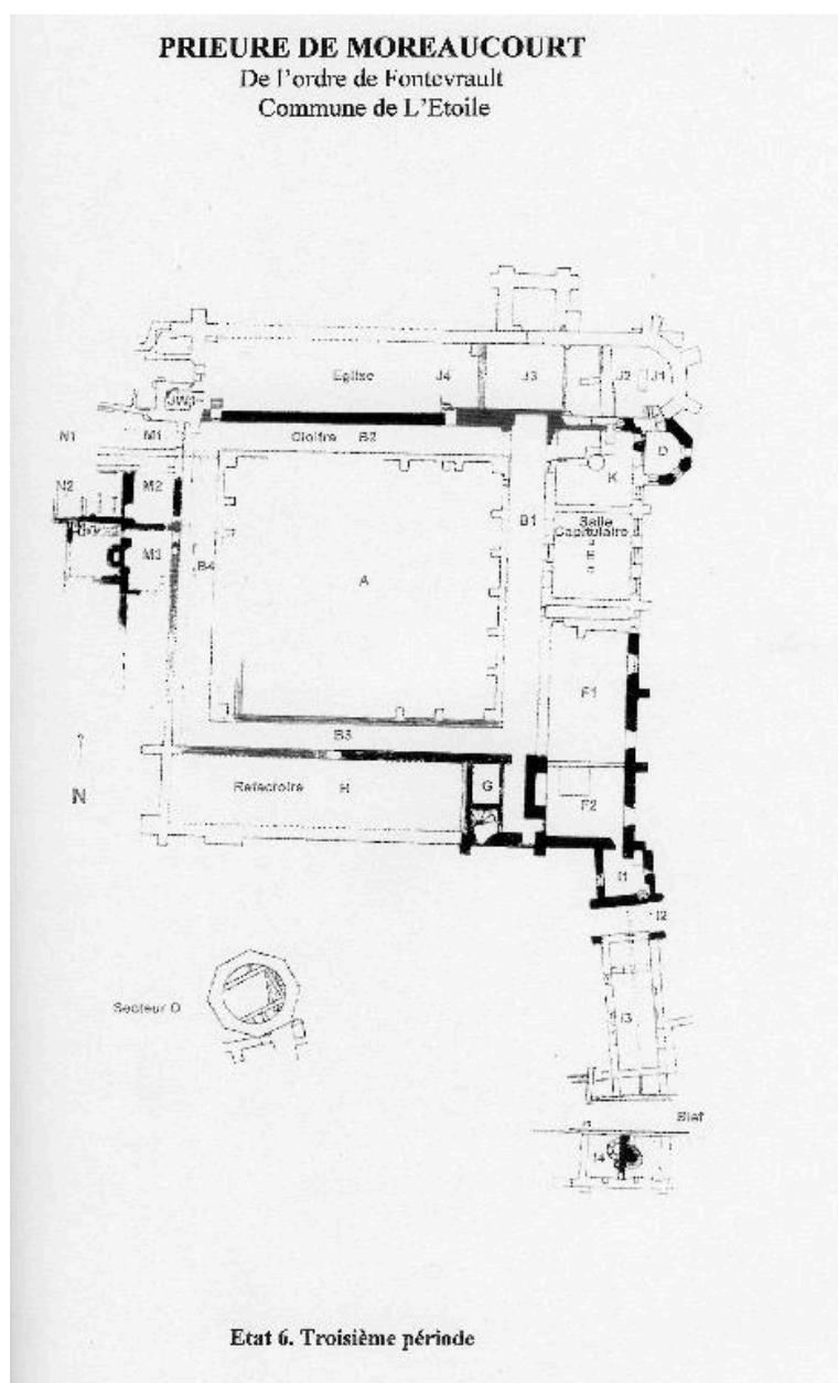
Plan du prieuré, état VI (troisième période), 1495-1522 : restitution par Gérard Cahon (35 ans de recherche sur Moreaucourt).
