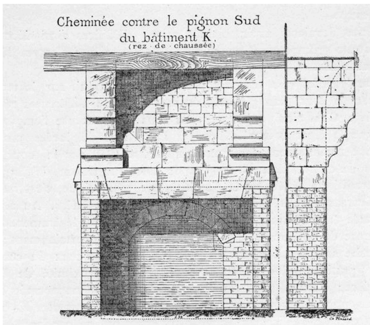
Cheminée du logis de l'ancienne ferme d'après Charles Pinsard (In : La Picardie historique et monumentale).
