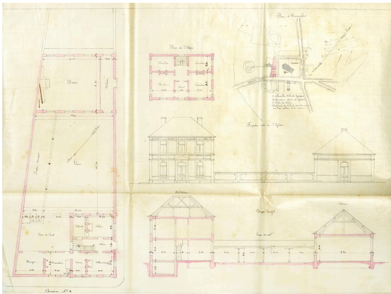
Plan d'ensemble, relevés et coupes de l'école de garçons de Zuytpeene, 1881 (AD Nord).
