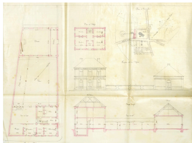
Plan d'ensemble, relevés et coupes de l'école de garçons de Zuytpeene, 1881 (AD Nord). Repro. Delphine Volto Jourdan IVR32_20255900059NUCA
