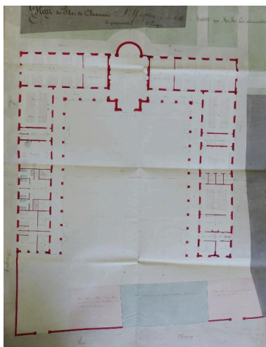
Projet de reconstruction de l'hôtel-Dieu. Plan du rez-de- chaussée, Daullé architecte, 1856 (AD Somme ; 99 O 2058). Phot. Barbedor Isabelle IVR22_20158006617NUCA
