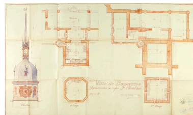
Ville de Bapaume - Reconstruction de l'église Saint-Nicolas - Clocher : plan ; élévation.
