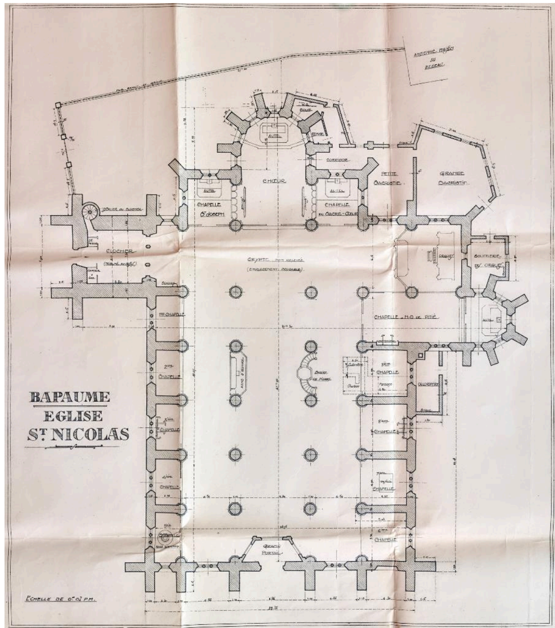
Bapaume - Église Saint-Nicolas. Ni daté ni signé. (AD Pas-de-Calais, 10R21/52) : plan de l'église avant-guerre.
