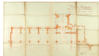
Ville de Bapaume - Reconstruction de l'église Saint-Nicolas : 1/2 plan côté tour. Dessin aquarellé, signé et daté, Eugène Bidard, 5 octobre 1929. (AD Pas-de-Calais, 20609/1). Phot. Pierre Thibaut IVR32_20216200152NUCA
