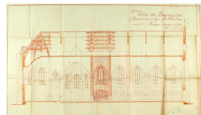
Ville de Bapaume - Reconstruction de l'église Saint-Nicolas : coupe longitudinale. Dessin aquarellé, signé et daté, Eugène Bidard, 5 octobre 1929. (AD Pas-de-Calais, 20609/1). Phot. Pierre Thibaut IVR32_20216200149NUCA
