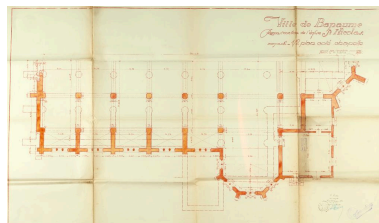
Ville de Bapaume - Reconstruction de l'église Saint-Nicolas : 1/2 plan côté chapelle. Dessin aquarellé, signé et daté, Eugène Bidard, 5 octobre 1929. (AD Pas-de-Calais, 20609/1). Phot. Pierre Thibaut IVR32_20216200150NUCA
