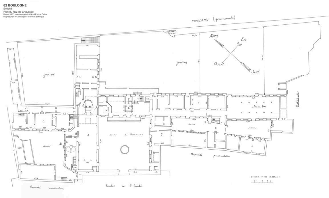
Plan du rez-de-chaussée, d'après un plan A.C. Boulogne -Services techniques.
