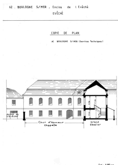
Façade de la chapelle de la cour d'honneur, d'après un tirage de plan, non daté, non signé (A.C. Boulogne- sur-Mer, services techniques).
