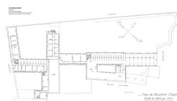
Plan du second étage, d'après un plan A.C. Boulogne -Services techniques. Repro. Eddy Stein, Phot. Eddy Stein IVR31_20146202734NUC
