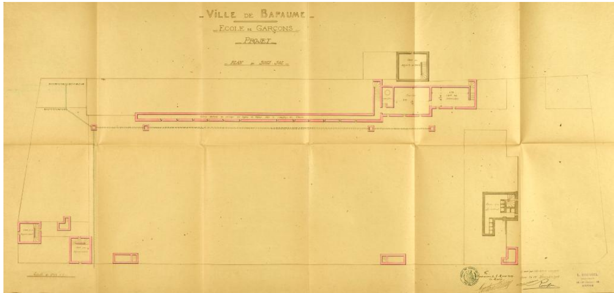
Ville de Bapaume, École de garçons - projet. Dessin aquarellé plan du sous-sol. Signé et daté L. Roussel, 15 décembre 1908 et 8 mars 1909. (AD Pas-de-Calais, 20612/1).
