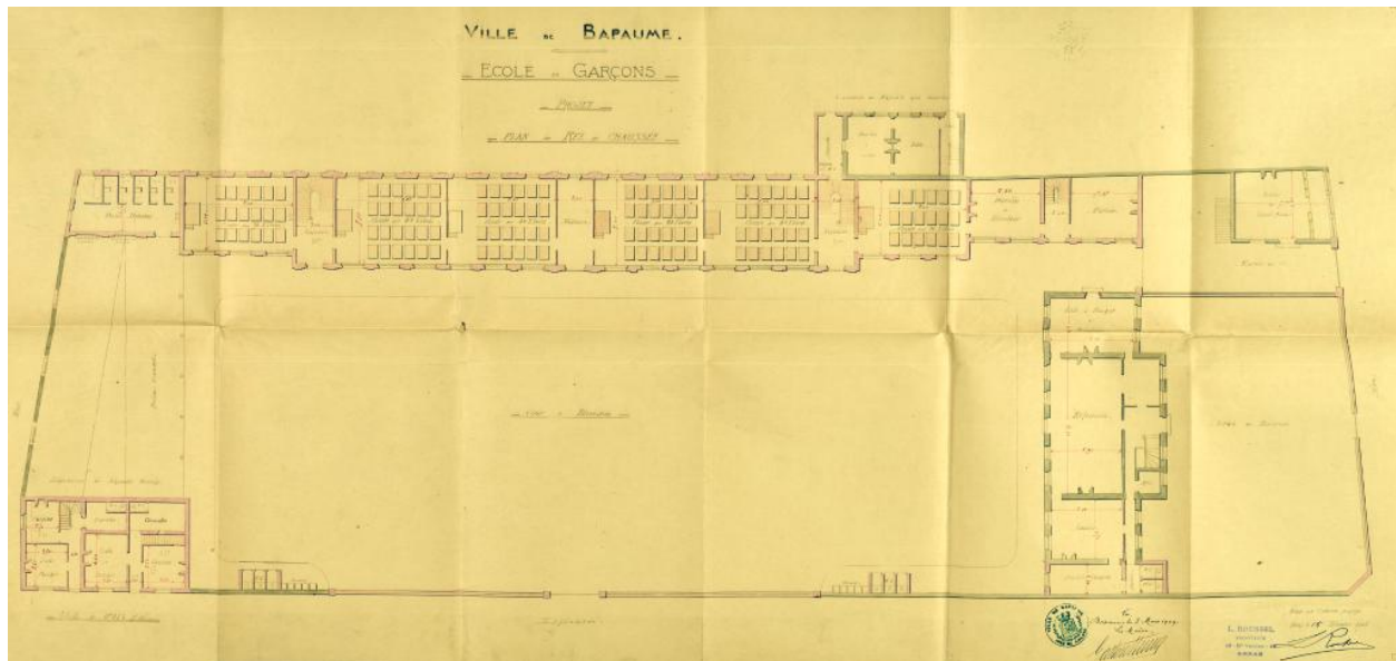
Ville de Bapaume, École de garçons - projet. Dessin aquarellé plan du rez-de-chaussée. Signé et daté L. Roussel, 15 décembre 1908 et 8 mars 1909. (AD pas-de-Calais, 20612/1).
