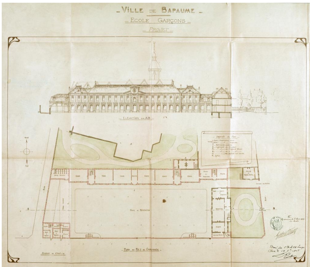
Ville de Bapaume, École de garçons - projet. Dessin aquarellé : élévation de la façade principale ; plan de situation. Signé et daté L. Roussel, 15 décembre 1908 et 8 mars 1909. (AD Pas-de-Calais, 20612/1).
