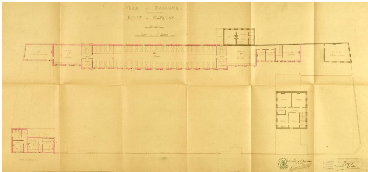
Ville de Bapaume, École de garçons - projet. Dessin aquarellé plan du premier étage. Signé et daté L. Roussel, 15 décembre 1908 et 8 mars 1909. (AD Pas-de-Calais, 20612/1).
