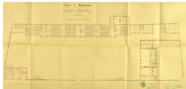
Ville de Bapaume, École de garçons - projet. Dessin aquarellé plan du rez-de-chaussée. Signé et daté L. Roussel, 15 décembre 1908 et 8 mars 1909. (AD pas-de-Calais, 20612/1). Phot. Pierre Thibaut IVR32_20216200301NUCA
