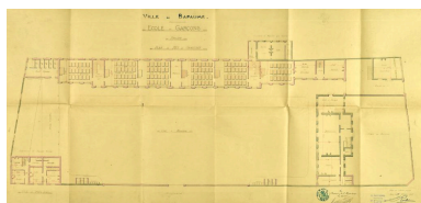
Ville de Bapaume, École de garçons - projet. Dessin aquarellé plan du rez-de-chaussée. Signé et daté L. Roussel, 15 décembre 1908 et 8 mars 1909. (AD pas-de-Calais, 20612/1). Phot. Thibaut Pierre (reproduction) IVR32_20216200301NUCA
