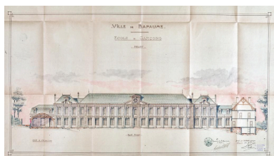
Ville de Bapaume, École de garçons - projet. Dessin aquarellé de la façade principale. Signé et daté L. Roussel, 15 octobre 1908 et 8 mars 1909. (AD Pas-de-Calais, 20612/1). Phot. Thibaut Pierre (reproduction) IVR32_20216200298NUCA
