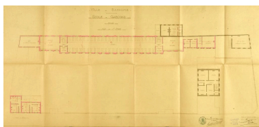
Ville de Bapaume, École de garçons - projet. Dessin aquarellé plan du premier étage. Signé et daté L. Roussel, 15 décembre 1908 et 8 mars 1909. (AD Pas-de-Calais, 20612/1). Phot. Thibaut Pierre (reproduction) IVR32_20216200300NUCA
