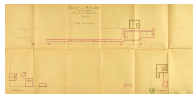
Ville de Bapaume, École de garçons - projet. Dessin aquarellé plan du sous-sol. Signé et daté L. Roussel, 15 décembre 1908 et 8 mars 1909. (AD Pas-de-Calais, 20612/1). Phot. Thibaut Pierre (reproduction) IVR32_20216200302NUCA
