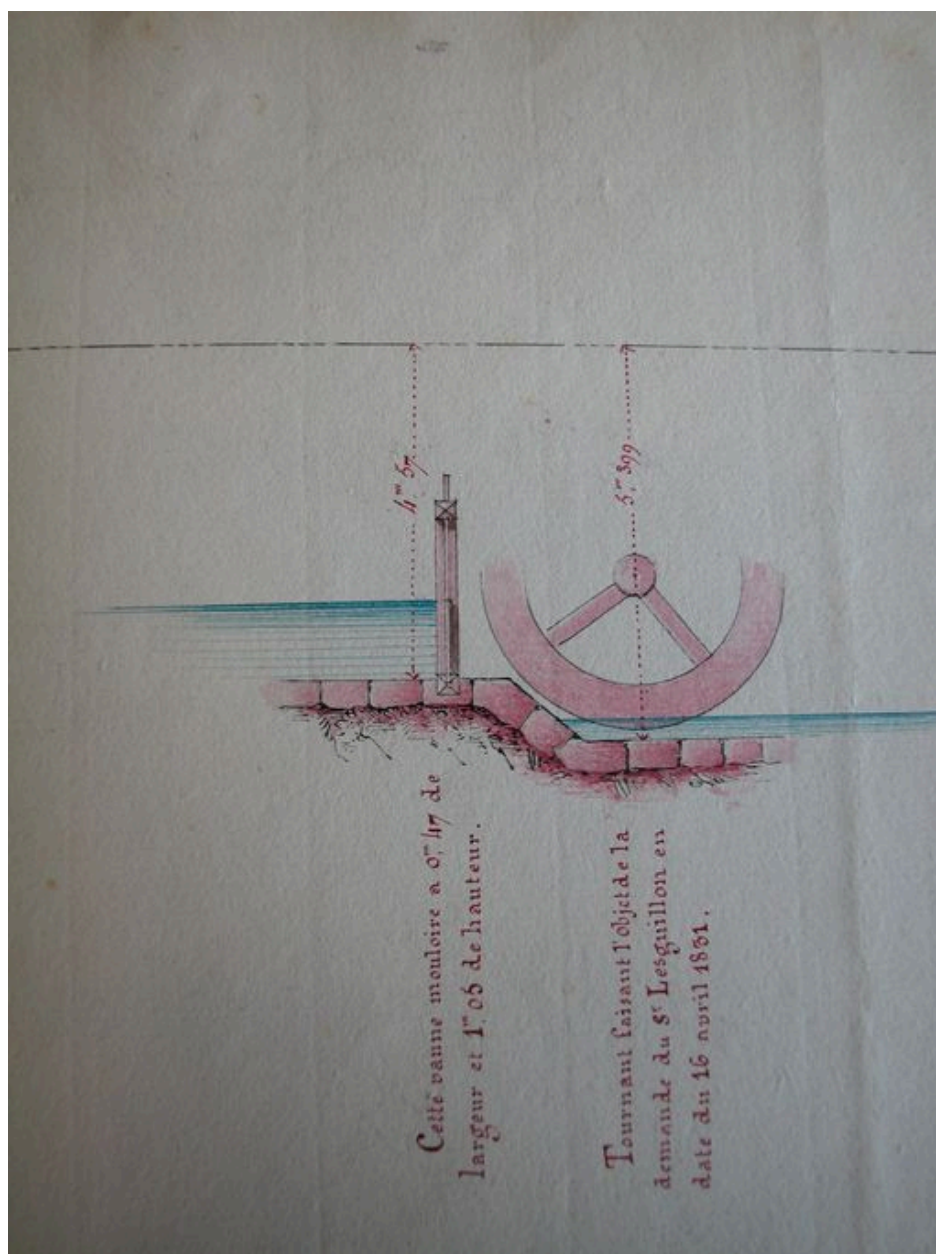
Profil de la seconde roue du moulin Lesguillon, devant faire l'objet de modifications, 1er décembre 1831.
