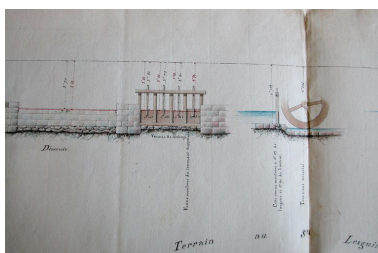
Profil de l'une des roues hydrauliques et du vannage de décharge du moulin Lesguillon, 1831.
