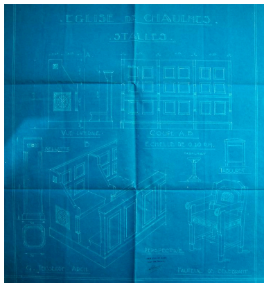
Projet de stalles, fauteuil de célébrant, tabouret par Godefroy Teisseire (AD Somme ; 99 O 1122). Phot. Gilles-Henri Bailly (reproduction) IVR22_20158005247NUCA
